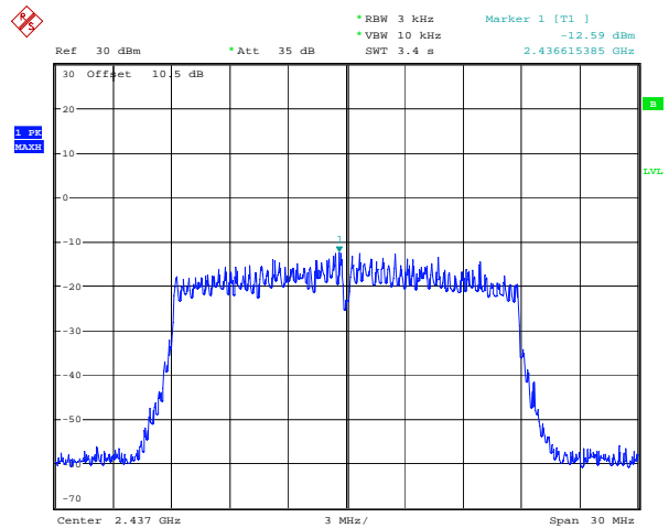
802.11n20_2437MHz
