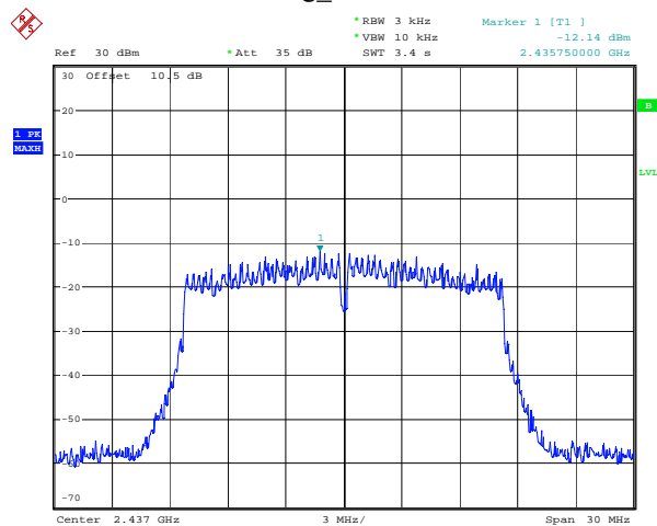
802.11g_2437MHz
