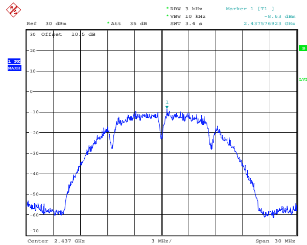
802.11b_2437MHz
