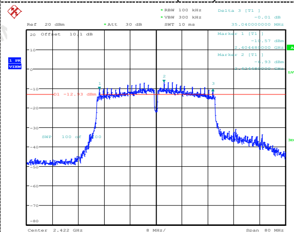
802.11n(HT40)
