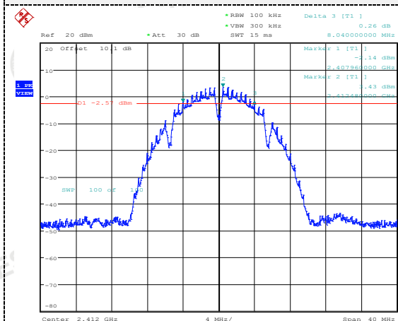
802.11b
