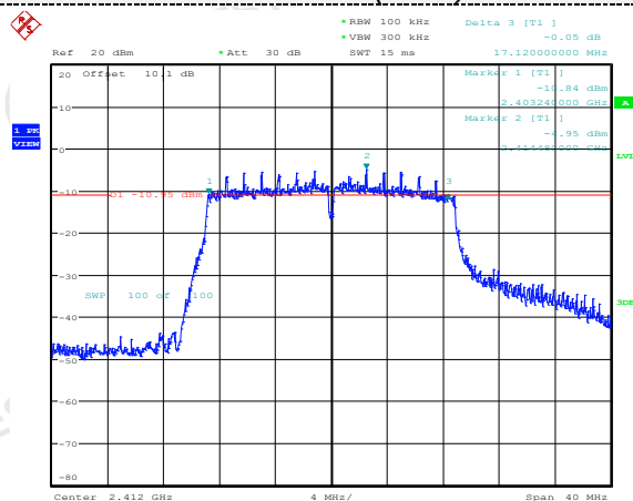
802.11n(HT20)
