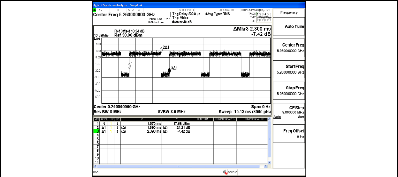
11AC20MIMO_Ant2_5260
