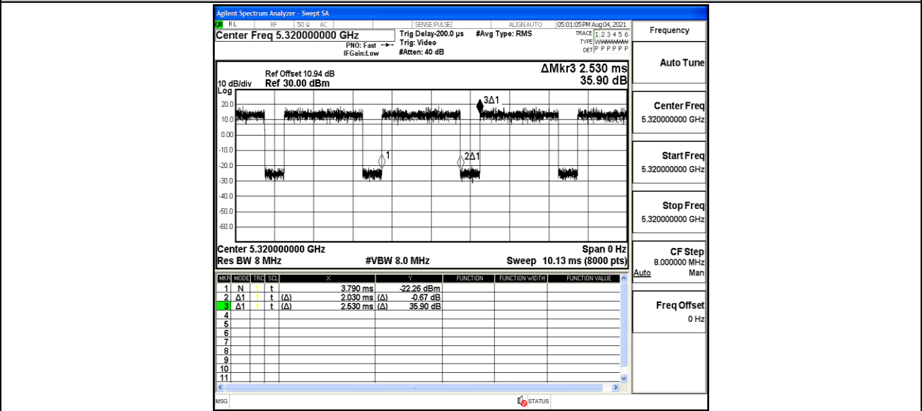
11A_Ant2_5320
