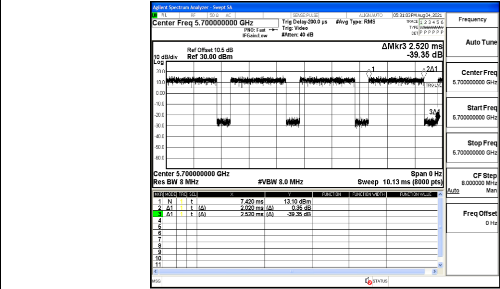
11A_Ant2_5700
