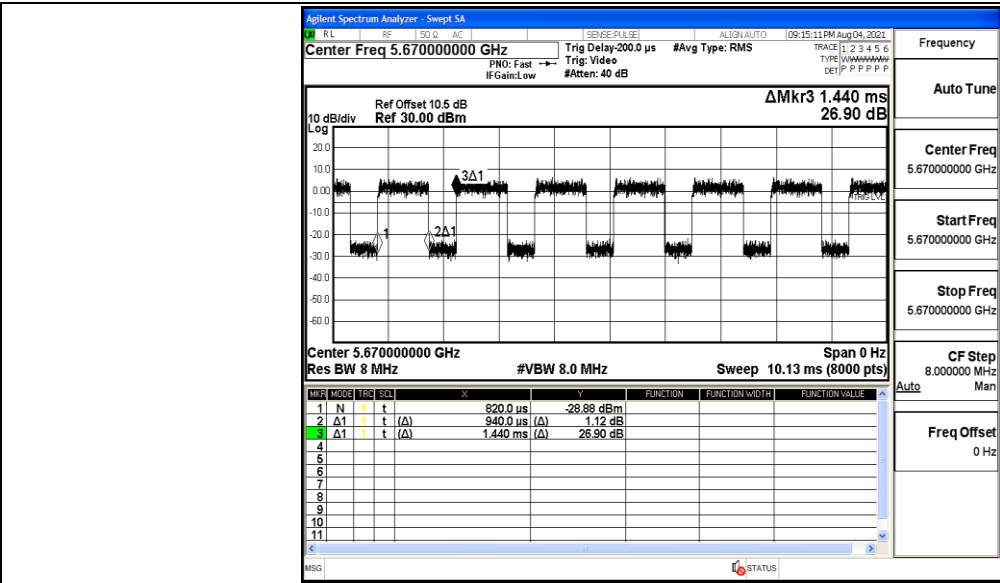
11AC40MIMO_Ant2_5670
