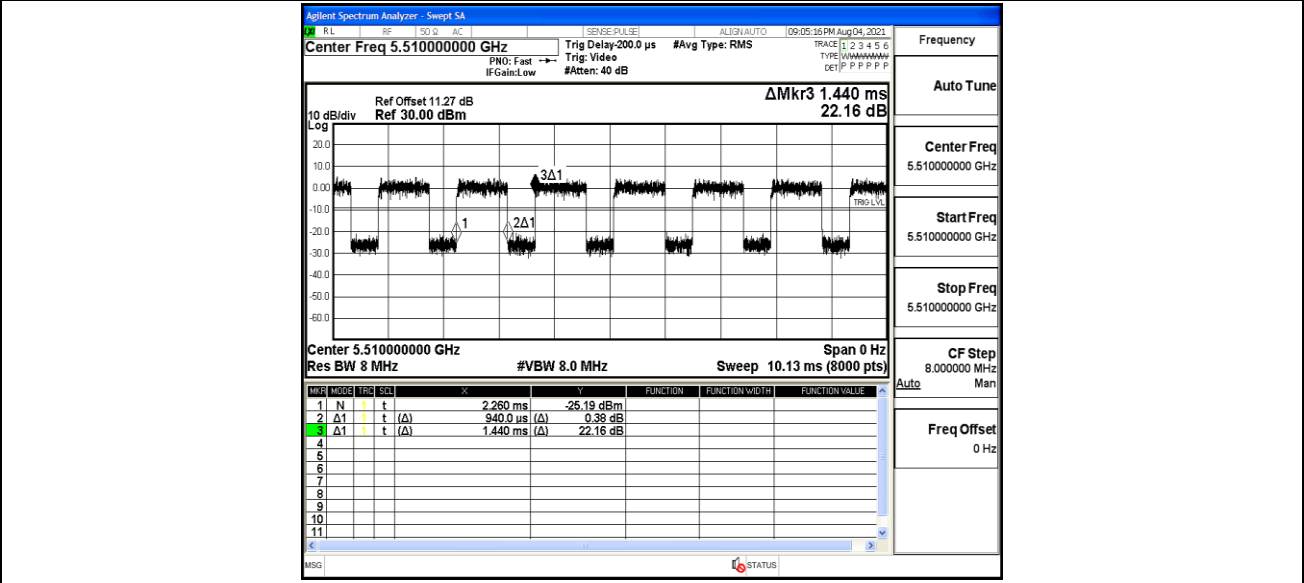
11AC40MIMO_Ant2_5510
