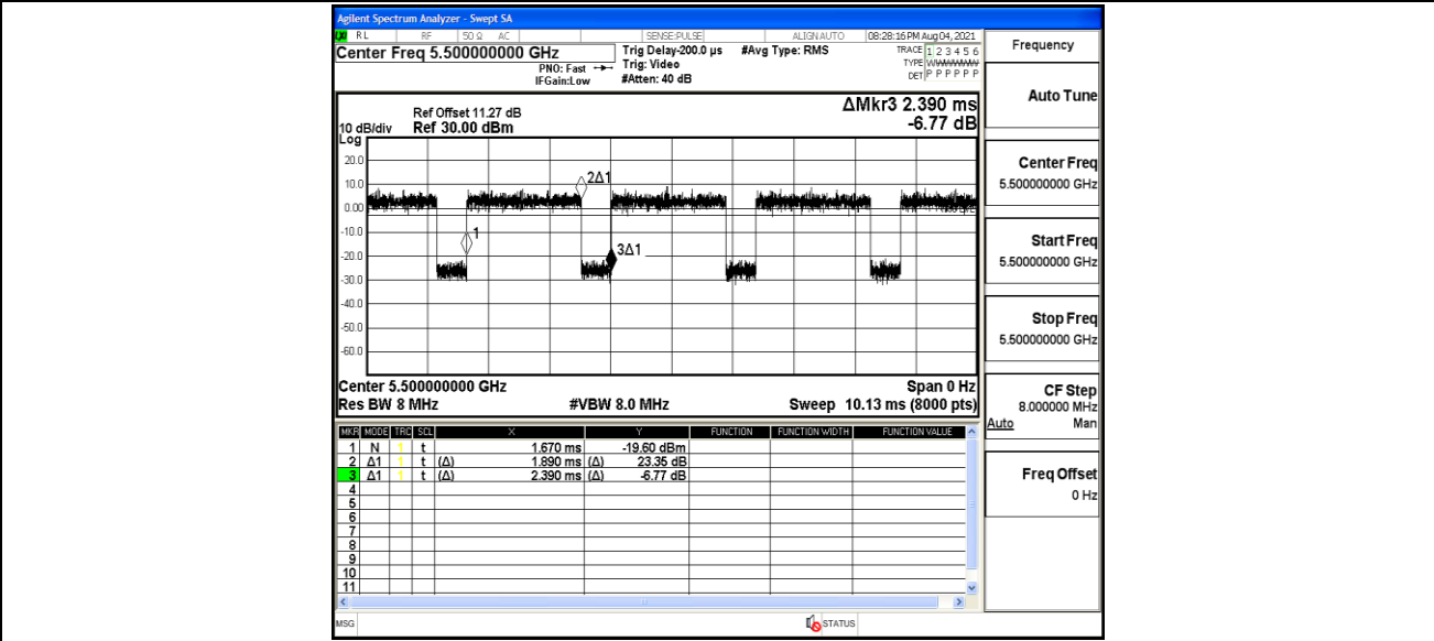
11AC20MIMO_Ant2_5500
