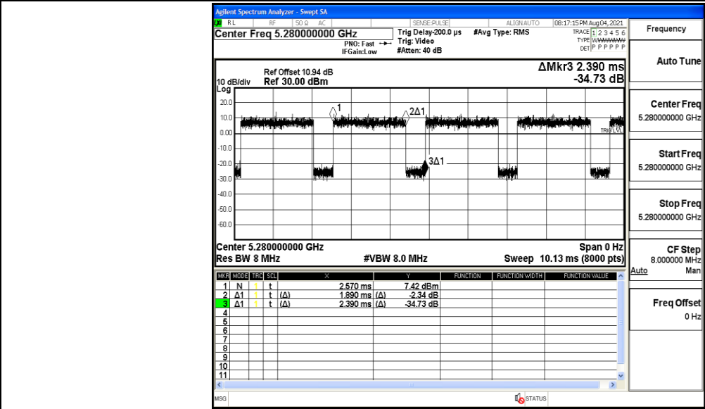
11AC20MIMO_Ant2_5280
