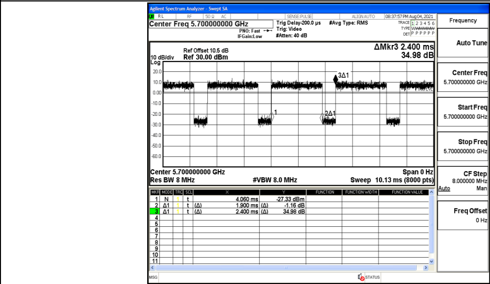
11AC20MIMO_Ant2_5700
