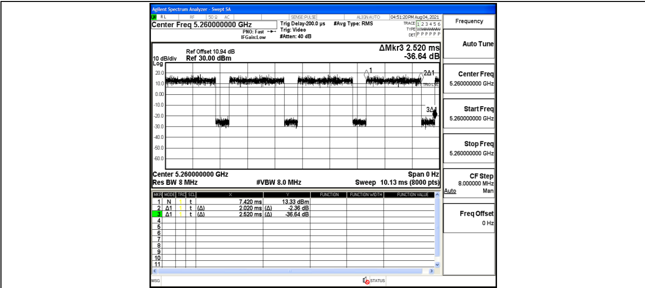
11A_Ant2_5260
