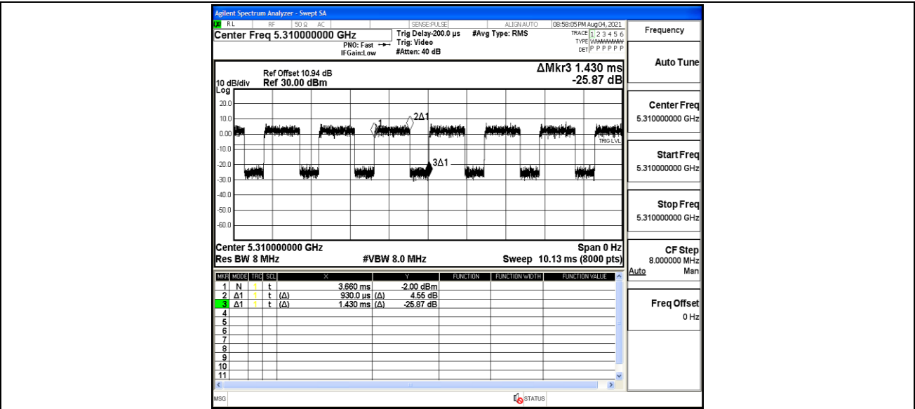
11AC40MIMO_Ant2_5310
