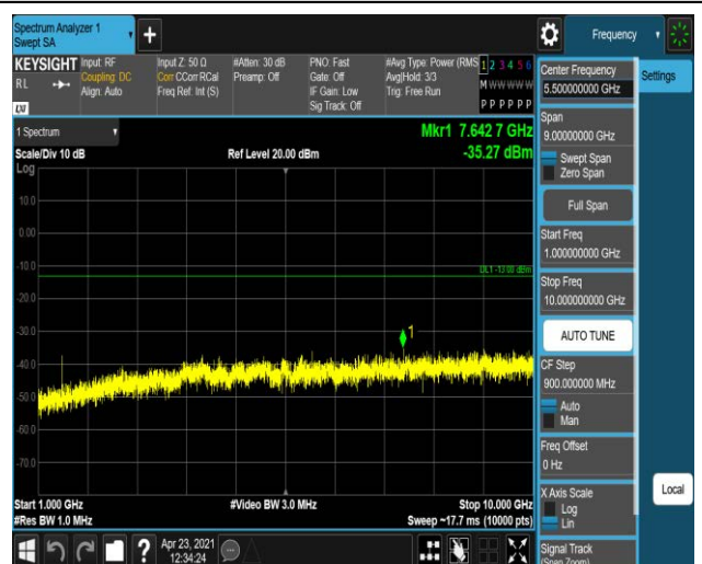
Band12-1.4MHz-16QAM-23017-1RB#0-Range2:1000~ 10000MHz
