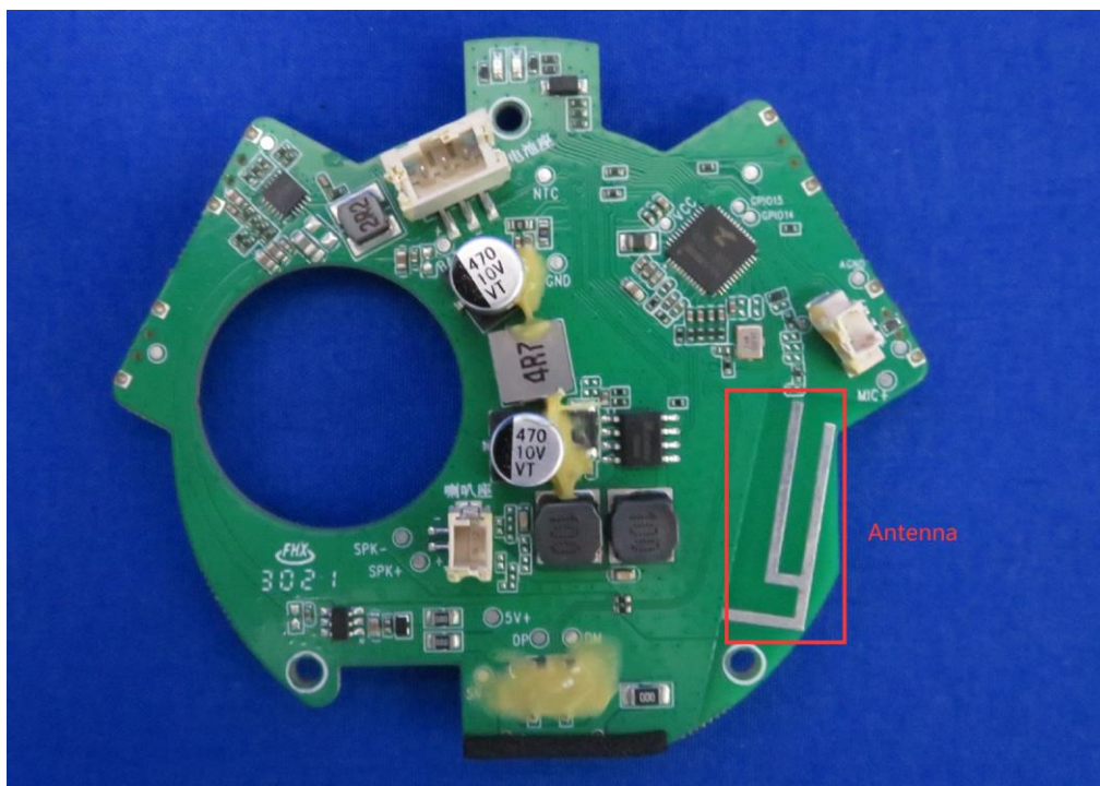
(8) EUT Photo
