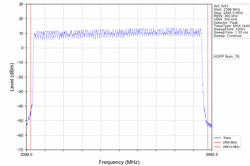
8DPSK_3DH5_HOPP_Ant1_NTNV
