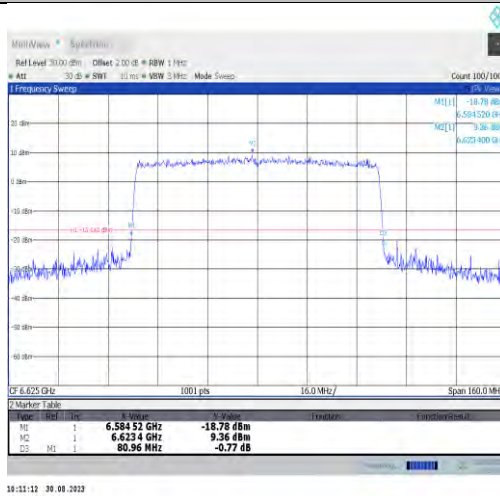
11ax80MIMO-Ant7-6625
