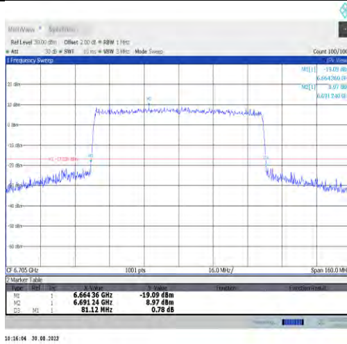
11ax80MIMO-Ant7-6705
