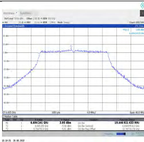
11x20MIMO-Ant7-6695-PASS
