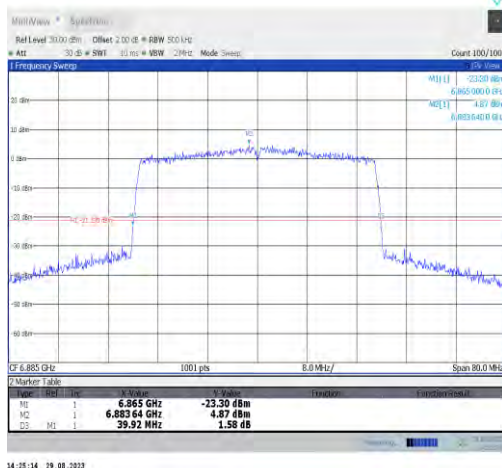
11ax40MIMO-Ant7-6885
