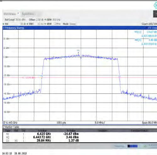
11ax40MIMO-Ant7-6445
