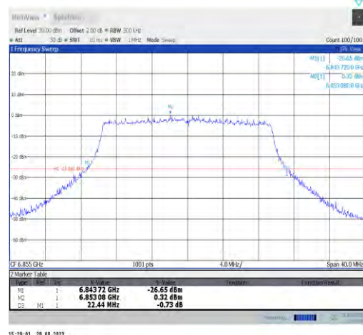
11ax20MIMO-Ant9-6855
