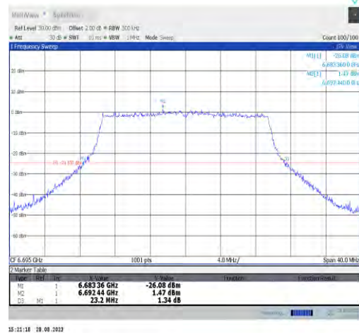
11ax20MIMO-Ant9-6695
