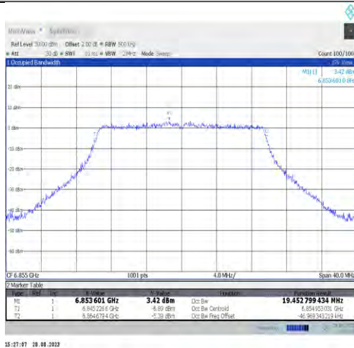
11x20MIMO-Ant7-6855-PASS
