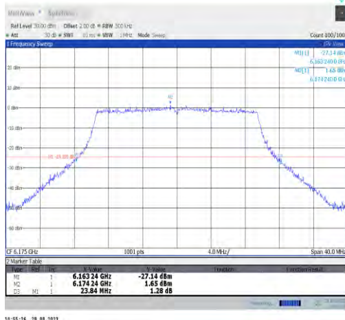
11ax20MIMO-Ant7-6175
