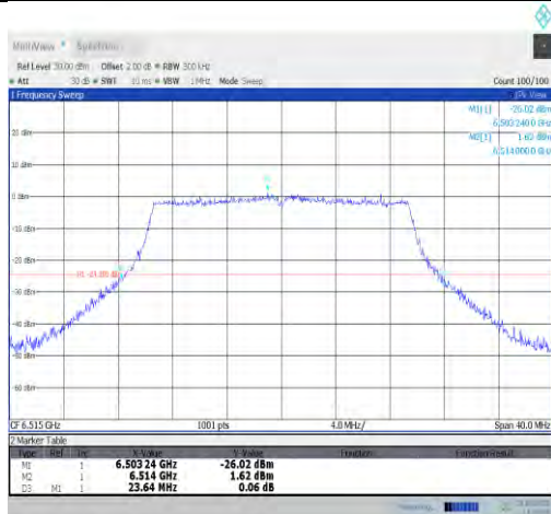
11ax20MIMO-Ant7-6515
