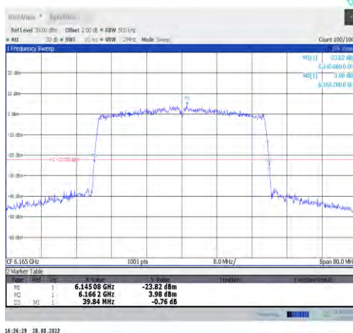
11ax40MIMO-Ant7-6165
