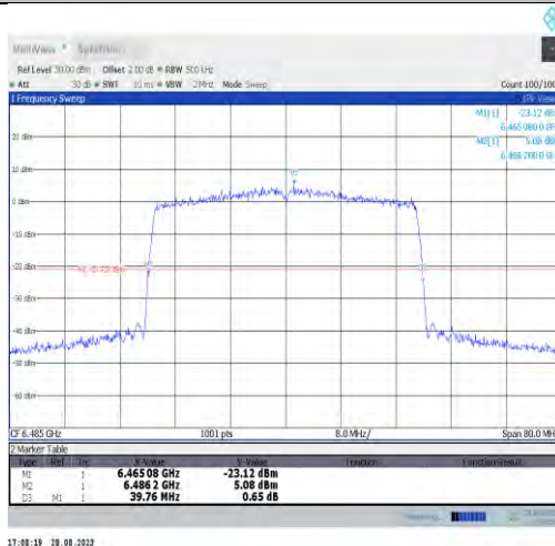
11ax40MIMO-Ant7-6485
