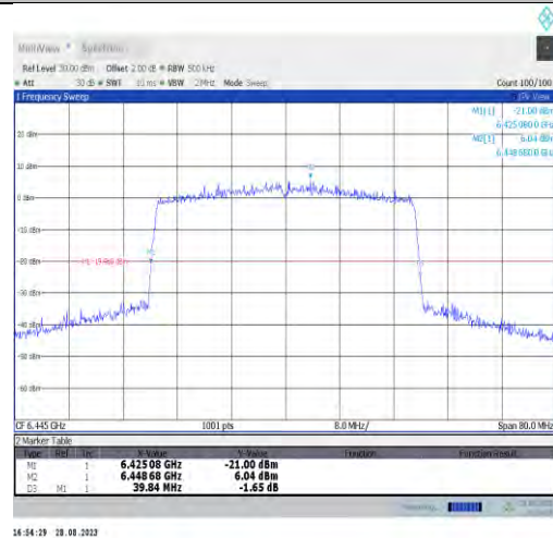
11ax40MIMO-Ant9-6445
