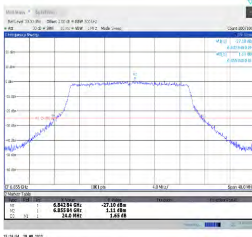
11ax20MIMO-Ant7-6855
