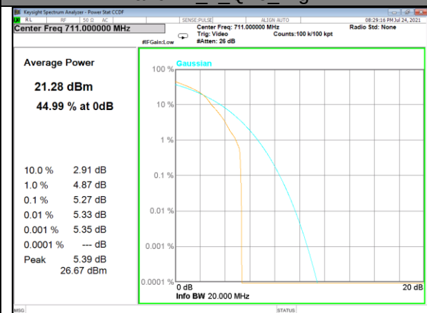
Band 17_1_Q16_High
