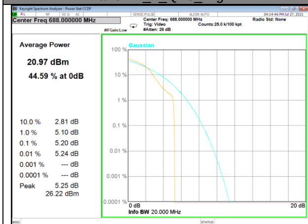
Band 71_1_Q16_High
