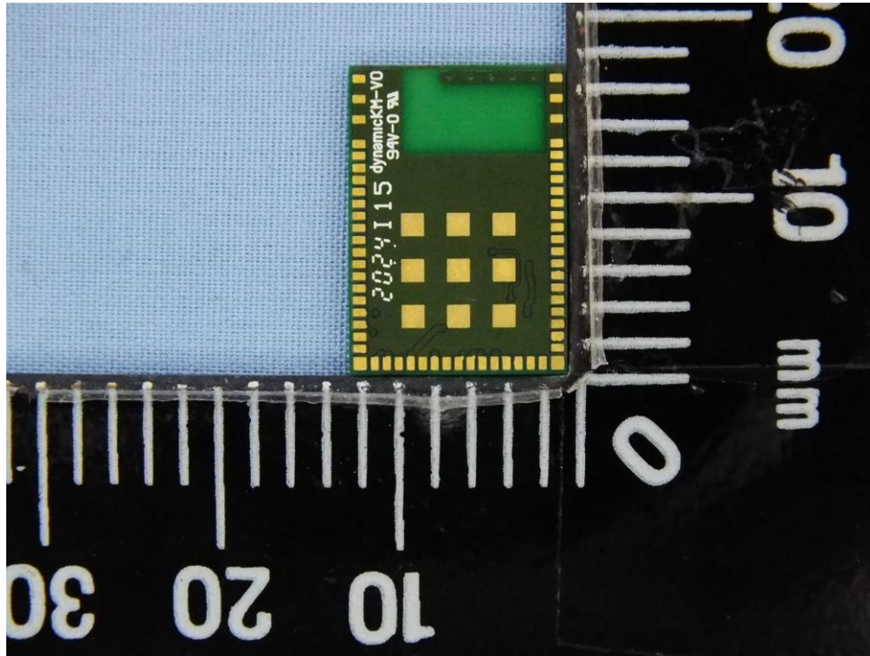
Part Number: 453-00047
