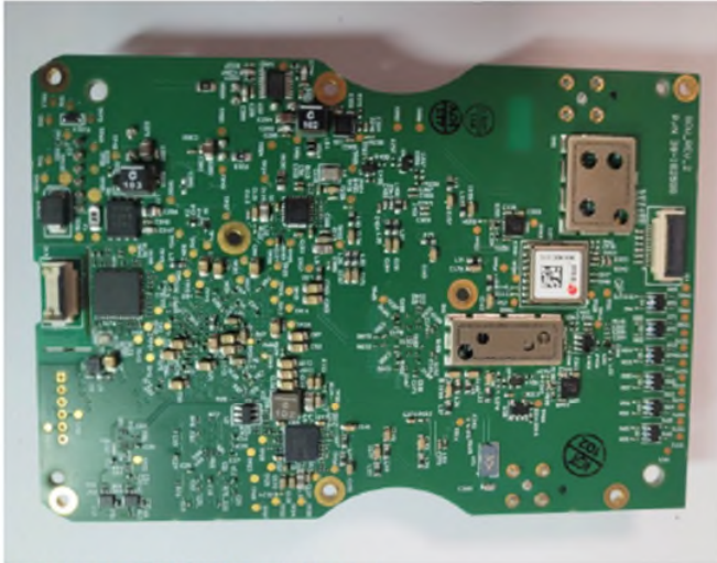
408060A T-TAC GCU Module Top View
