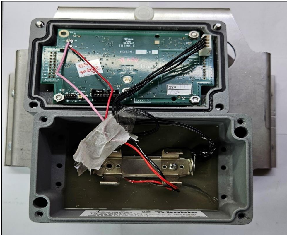
EUT Encloser Open
