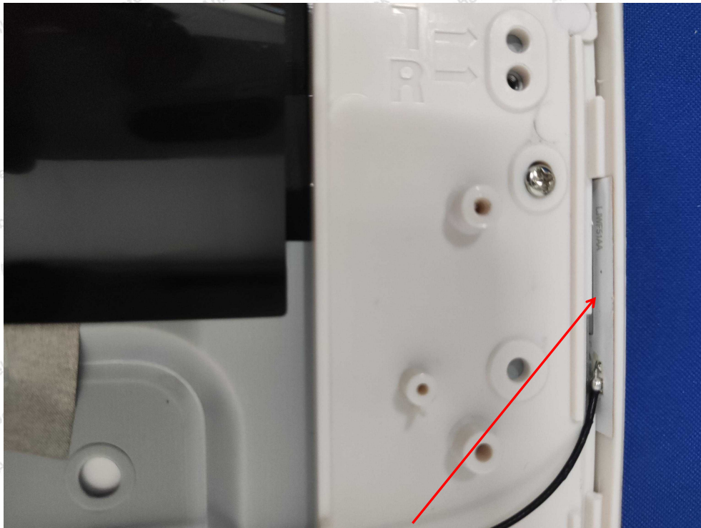
BLE&WiFi 2.4G&WiFi 5G ANT
