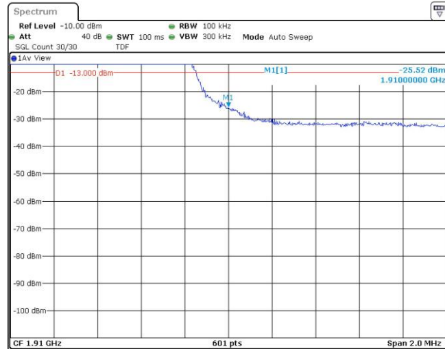
Band2-10MHz-QPSK-18650-1RB#0
