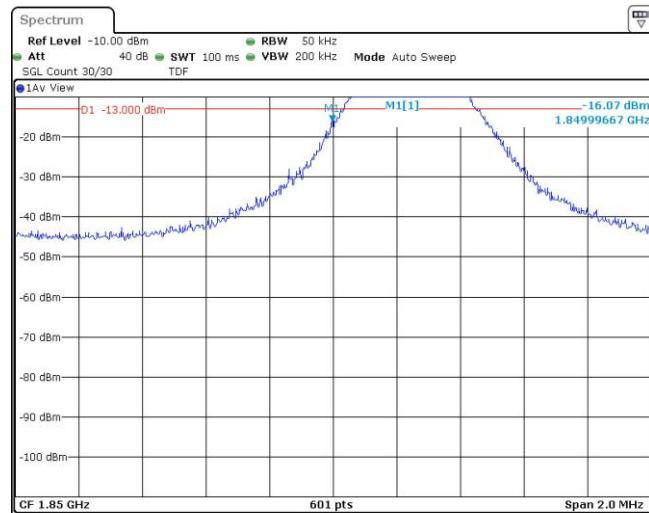
Band2-3MHz-QPSK-18615-1RB#14
