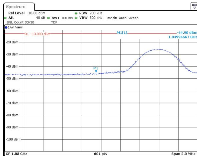
Band2-10MHz-QPSK-18650-25RB#0
