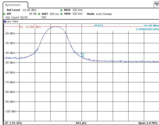
Band2-5MHz-QPSK-19175-1RB#24
