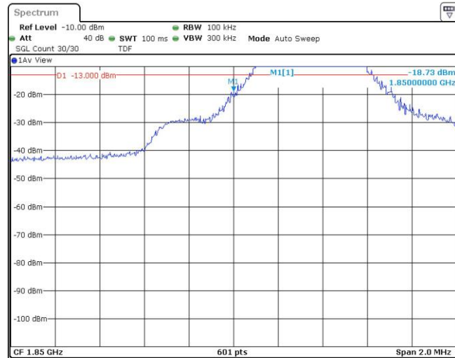
Band2-5MHz-QPSK-18625-1RB#24
