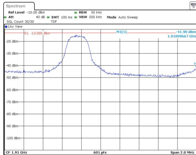
Band2-3MHz-QPSK-19185-1RB#14
