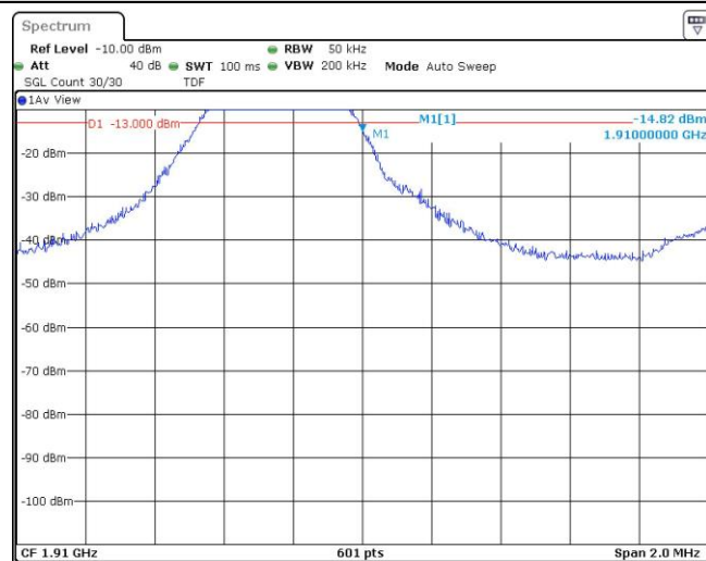
Band2-3MHz-QPSK-19185-15RB#0
