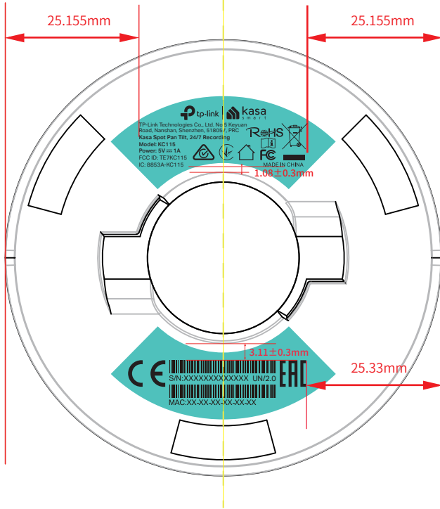
尺寸图
