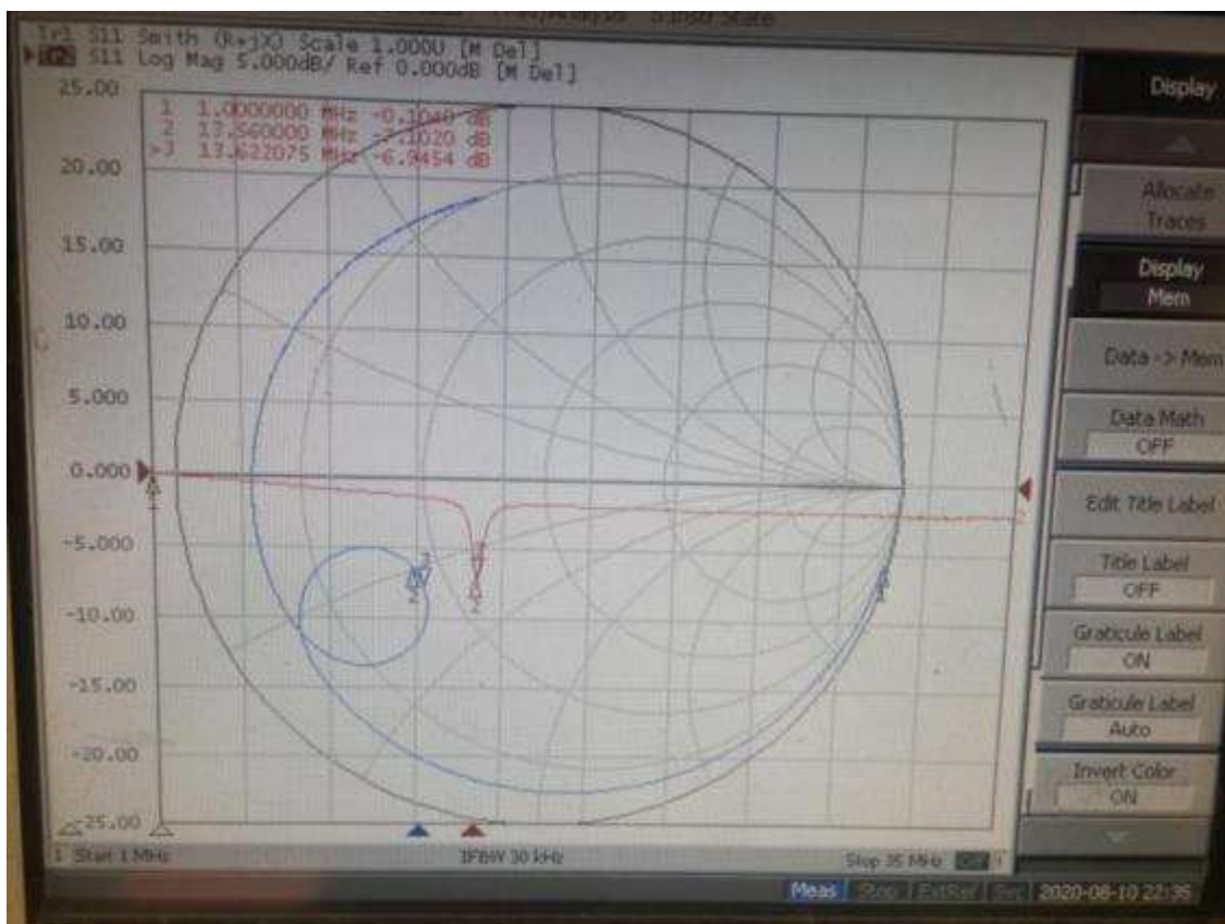
NFC antenna
