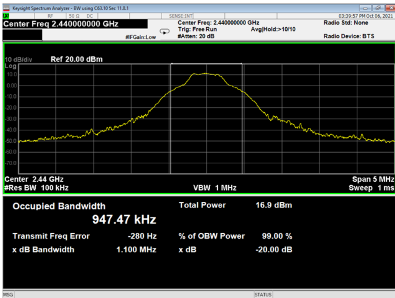
05 OBW-20dB, Mid.png
