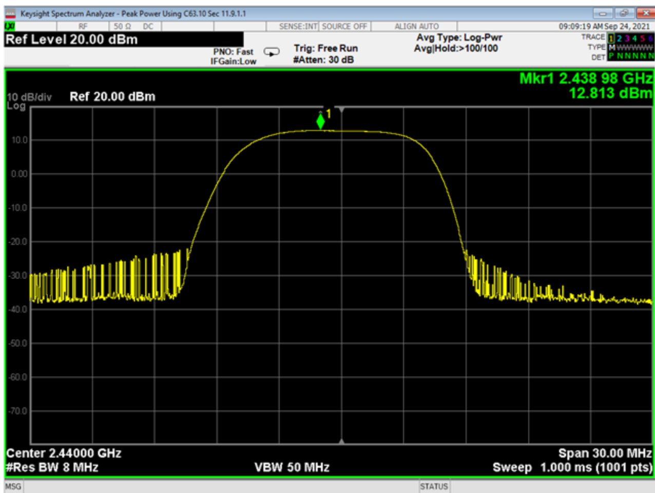
02 Pwr, Mid.png
