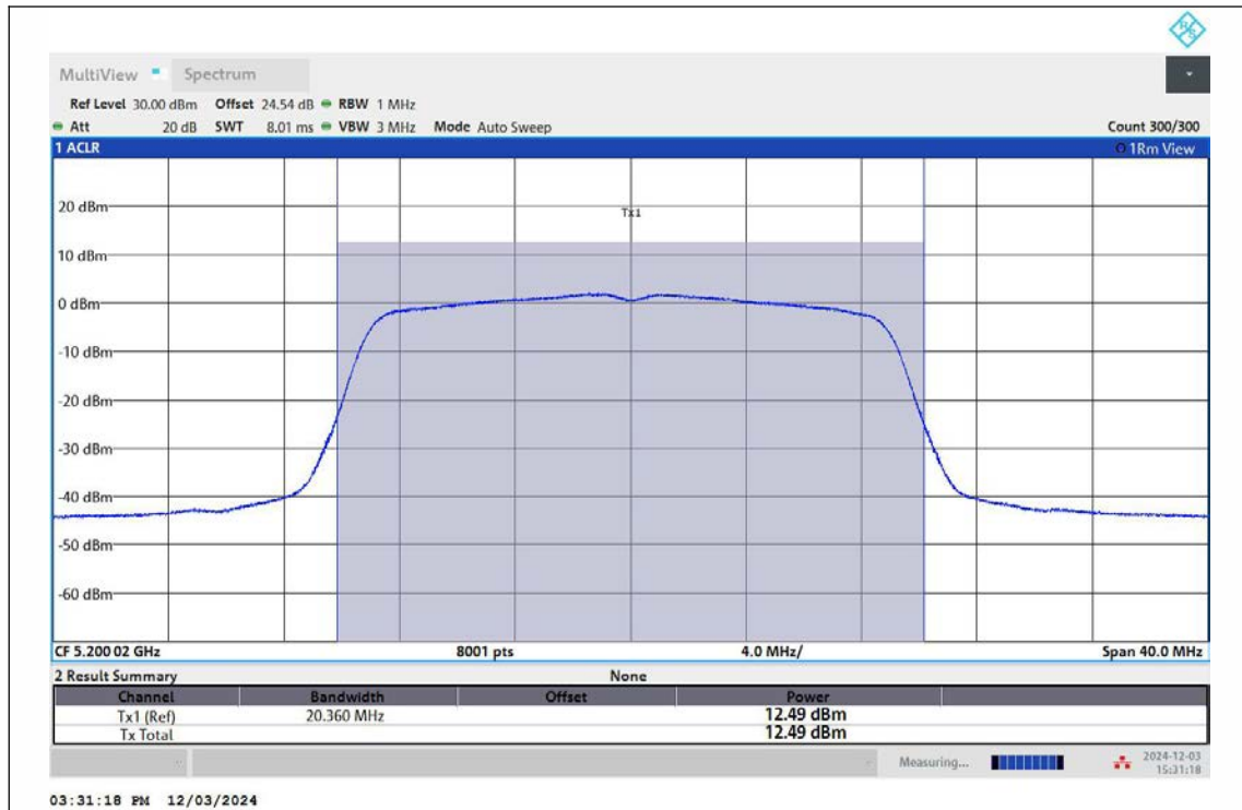
11N20MIMO-Ant1-5200-PASS
