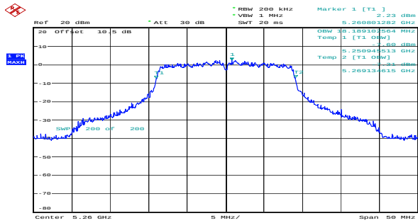
n20_5260MHz_Chain 0 18.189MHz
