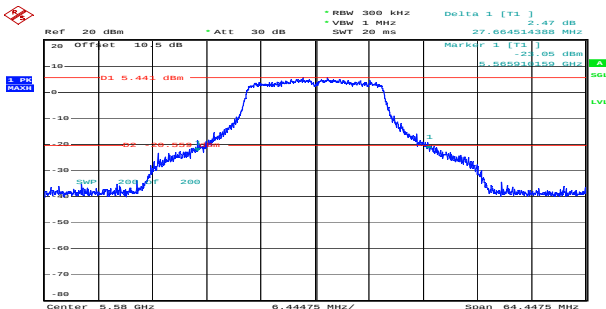
a_5580MHz_Chain 0 27.665MHz
