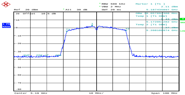
n40_5190MHz_Chain 0 36.058MHz
