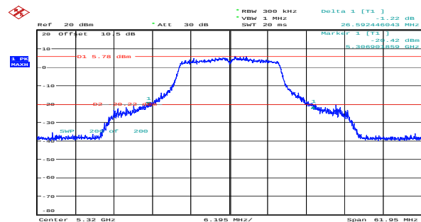
a_5320MHz_Chain 0 26.592MHz
