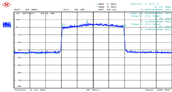
ax80 5210MHz RU Full Chain 0 76.960MHz
