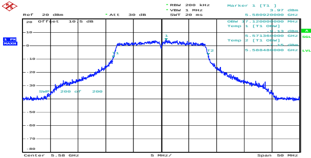
a_5580MHz_Chain 0 17.120MHz
