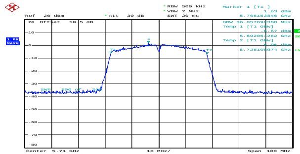
n40_5710MHz_Chain 0 36.058MHz
