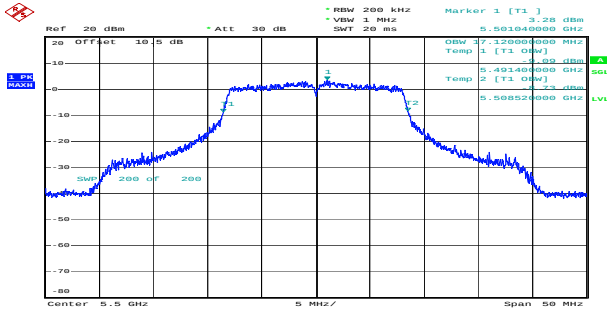
a_5500MHz_Chain 0 17.120MHz
