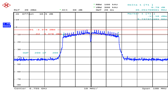
n40_5755MHz_Chain 0 35.252MHz
