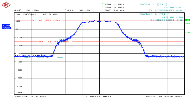
n20_5500MHz_Chain 0 37.276MHz
