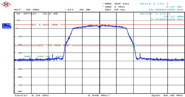
a_5240MHz_Chain 0 20.370MHz
