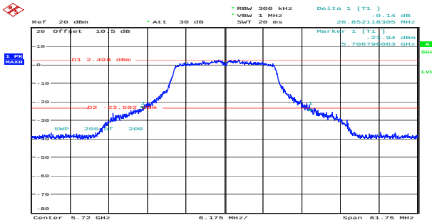
a_5720MHz_Chain 0 26.852MHz
