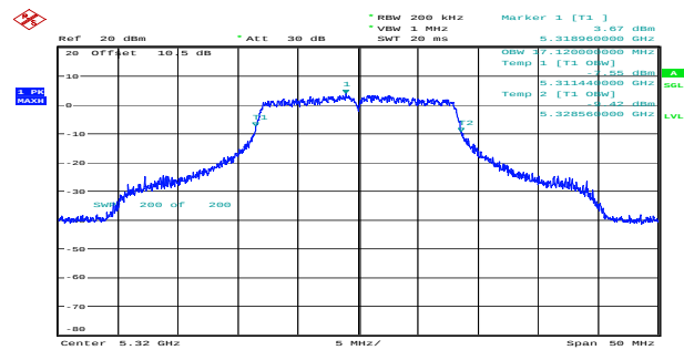
a_5320MHz_Chain 0 17.120MHz
