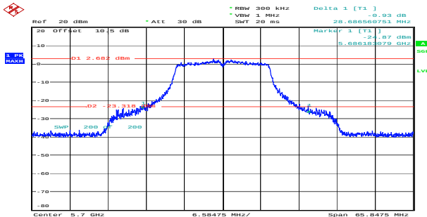
a_5700MHz_Chain 0 28.687MHz
