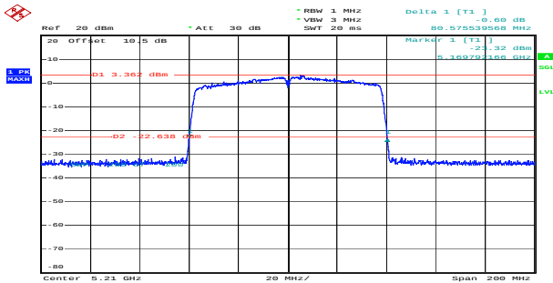
ac80_5210MHz_Chain 0 80.576MHz
