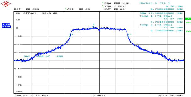
a_5720MHz_Chain 0 17.160MHz
