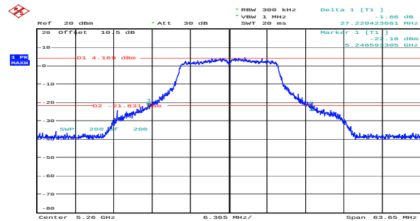
a_5260MHz_Chain 0 27.220MHz
