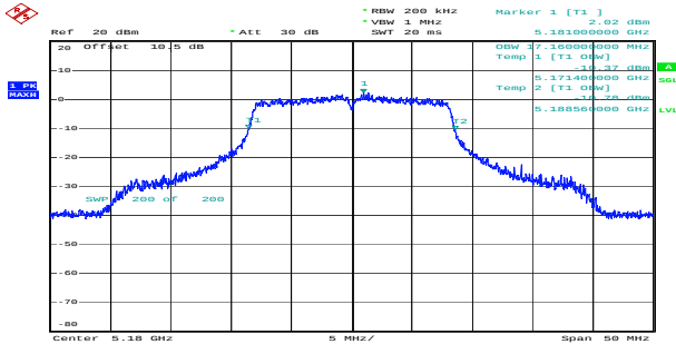
a_5180MHz_Chain 0 17.160MHz
