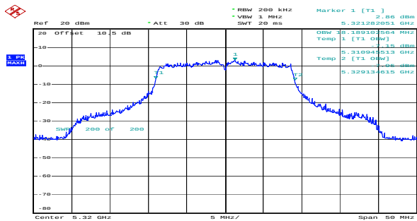
n20_5320MHz_Chain 0 18.189MHz
