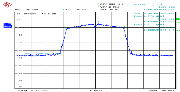
n40_5550MHz_Chain 0 36.058MHz
