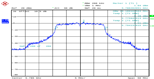
n20_5785MHz_Chain 0 18.189MHz
