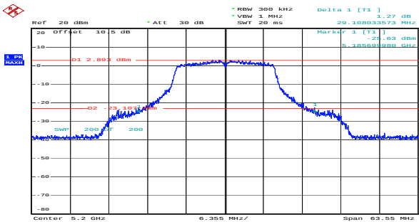
a_5200MHz_Chain 0 29.108MHz
