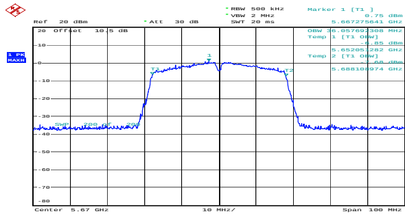
n40_5670MHz_Chain 0 36.058MHz
