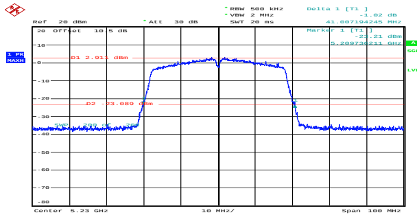
n40_5230MHz_Chain 0 41.007MHz
