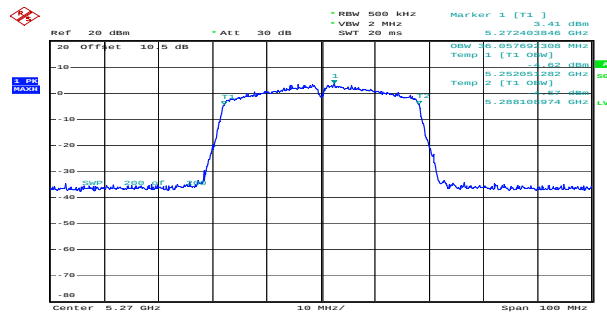
n40_5270MHz_Chain 0 36.058MHz
