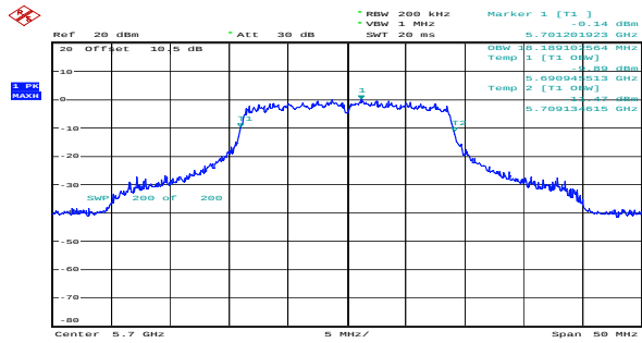
n20_5700MHz_Chain 0 18.189MHz
