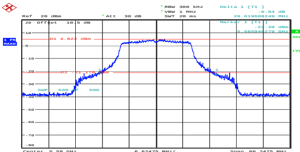
n20_5580MHz_Chain 0 29.020MHz
