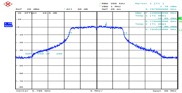
a_5785MHz_Chain 0 17.120MHz
