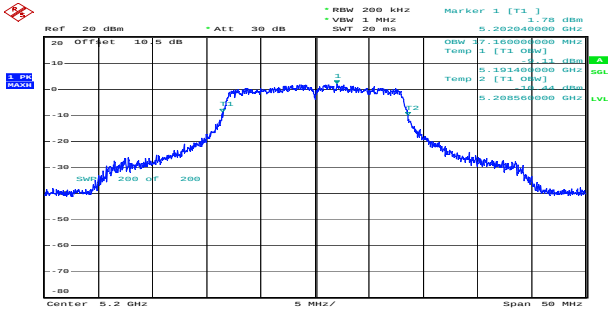
a_5200MHz_Chain 0 17.160MHz
