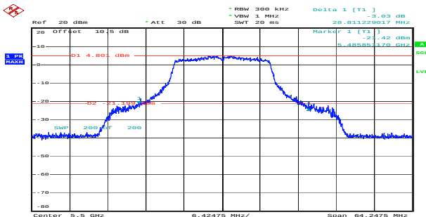
a_5500MHz_Chain 0 28.811MHz
