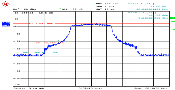
n20_5260MHz_Chain 0 28.898MHz
