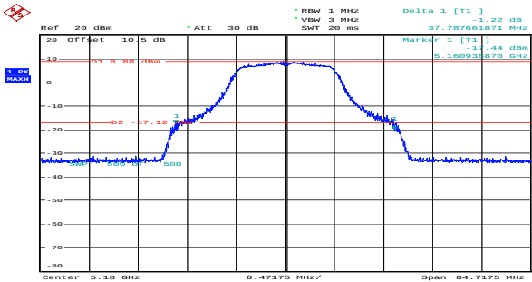
n20_5180MHz_Chain 0 37.788MHz
