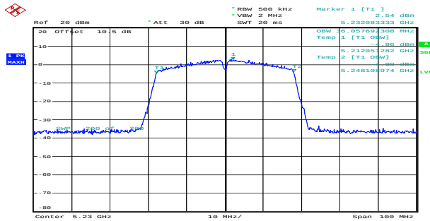
n40_5230MHz_Chain 0 36.058MHz
