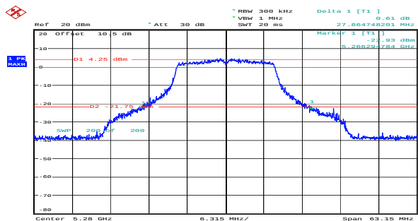
a_5280MHz_Chain 0 27.865MHz
