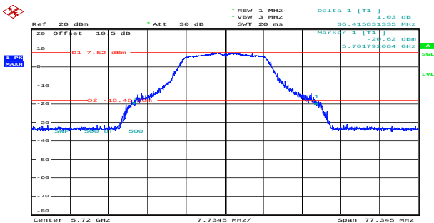
n20_5720MHz_Chain 0 36.416MHz
