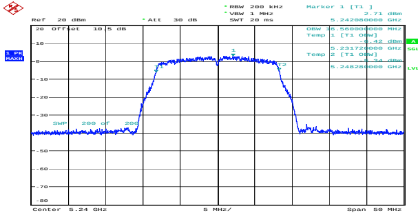
a_5240MHz_Chain 0 16.560MHz
