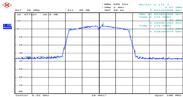
n40_5510MHz_Chain 0 36.058MHz
