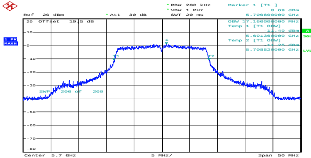
a_5700MHz_Chain 0 17.160MHz
