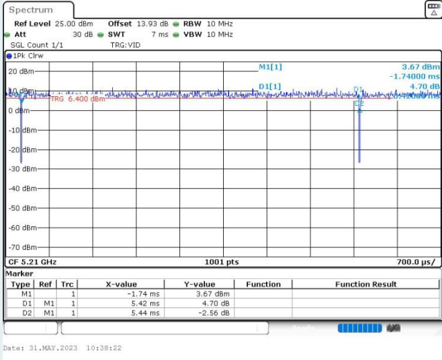
802.11ac VHT80_5210MHz
