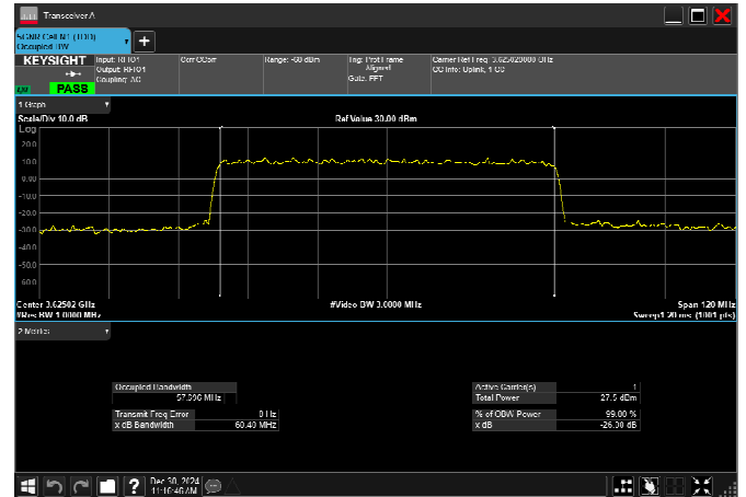
n77_2_70MHz_30kHz_3625MHz_DFT-s-OFDM \pi/2 BPSK_RB180@0 67.214MHz
