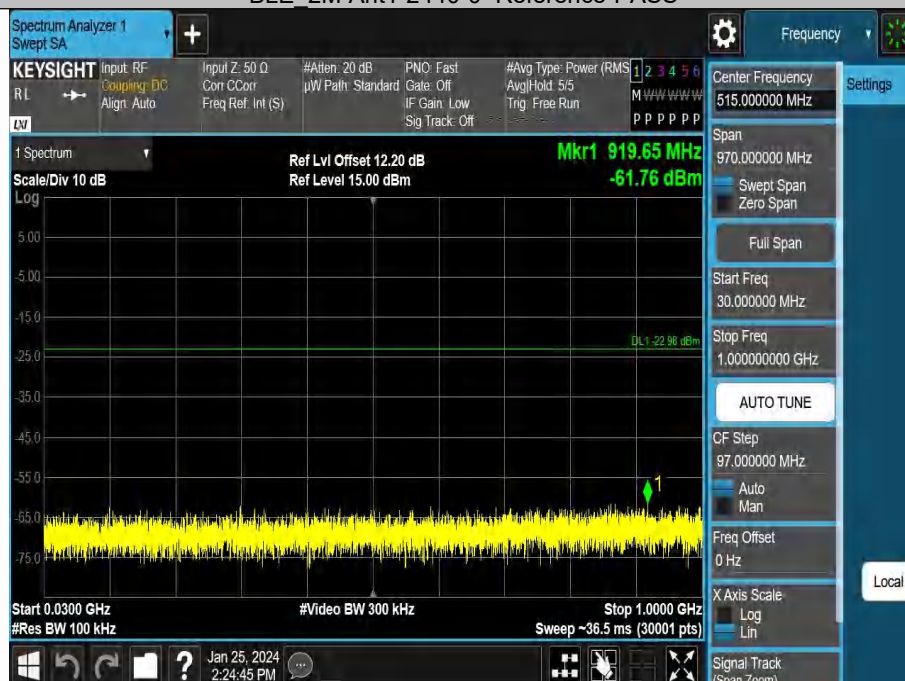
BLE_2M-Ant1-2440-30~1000-PASS
