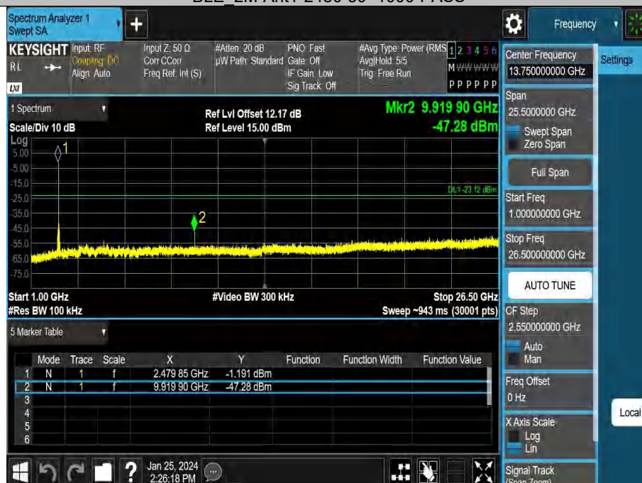
BLE 2M-Ant1-2480-1000~26500-PASS
