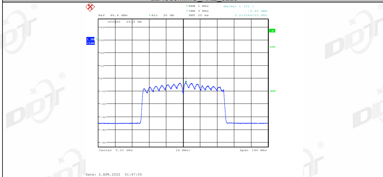
11AC80MIMO_Ant2_5210
