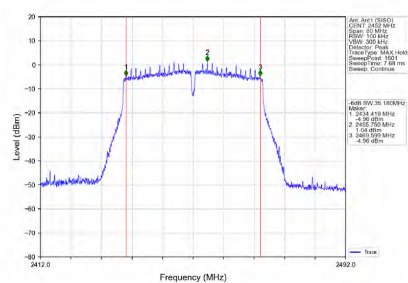
802.11n(HT40)_HCH_2452MHz_Ant1 (SISO)_NTNV
