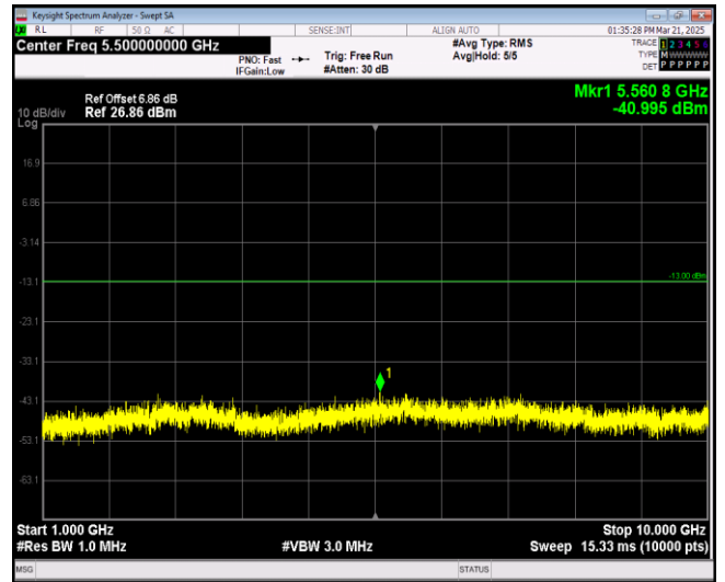
Band12-10MHz-QPSK-23060-1RB#0-Range2:1000~ 10000MHz
