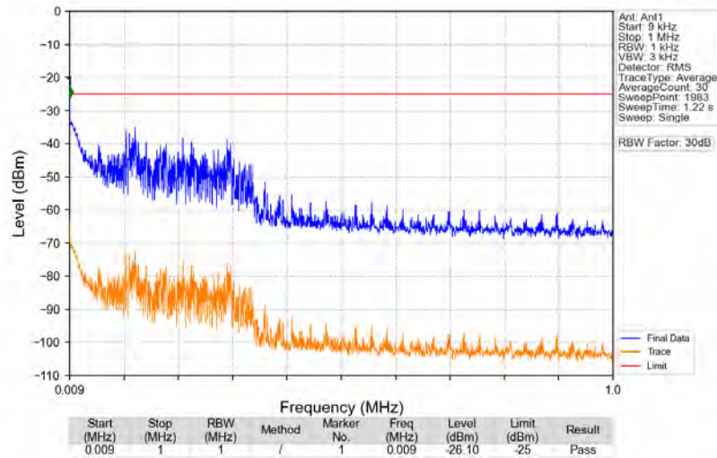
n41_30kHz_SISO_NTNV_60MHz_DFT-s-OFDM_QPSK_2526MHz_Edge_1RB_Left
