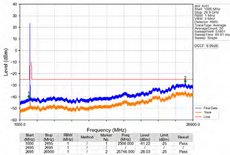
n41_30kHz_SISO_NTNV_70MHz_DFT-s-OFDM_PI/2_BPSK_2531.01MHz_Edge_1RB_Left
