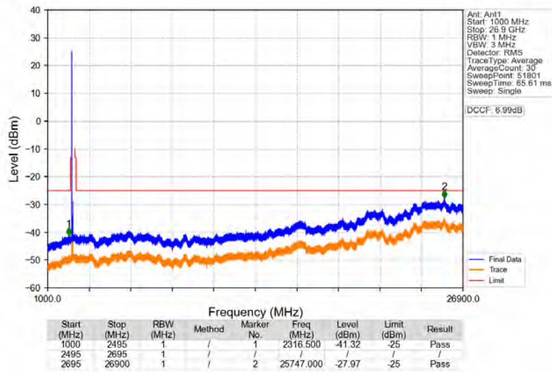
n41_30kHz_SISO_NTNV_80MHz_DFT-s-OFDM_PI/2_BPSK_2536.02MHz_Edge_1RB_Left
