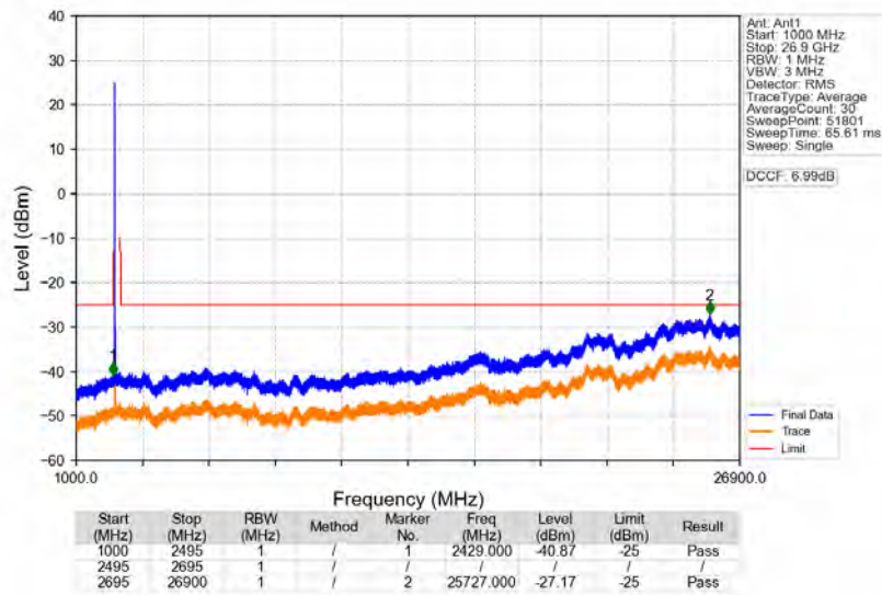
n41_30kHz_SISO_NTNV_50MHz_DFT-s-OFDM_PI/2_BPSK_2521.02MHz_Edge_1RB_Left
