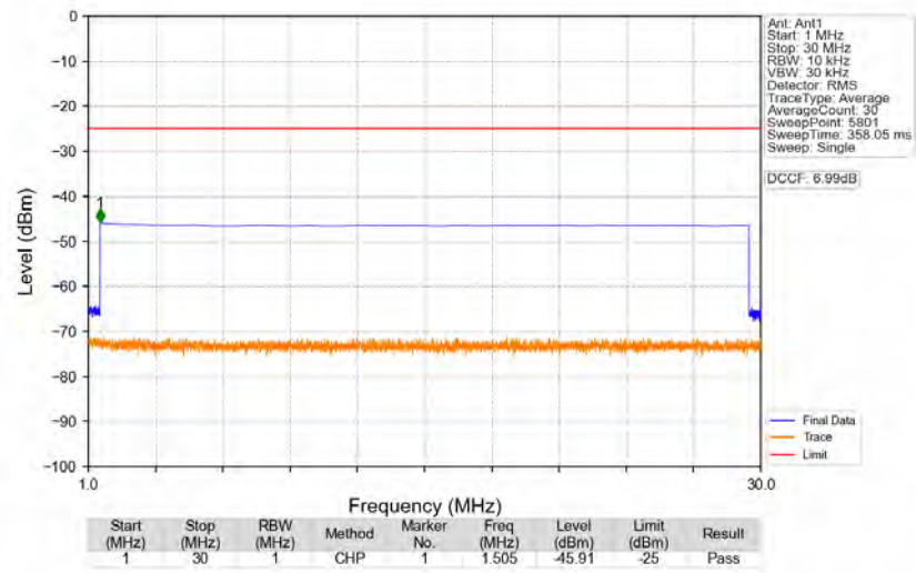
n41_30kHz_SISO_NTNV_60MHz_CP-OFDM_QPSK_2526MHz_Edge_1RB_Left
