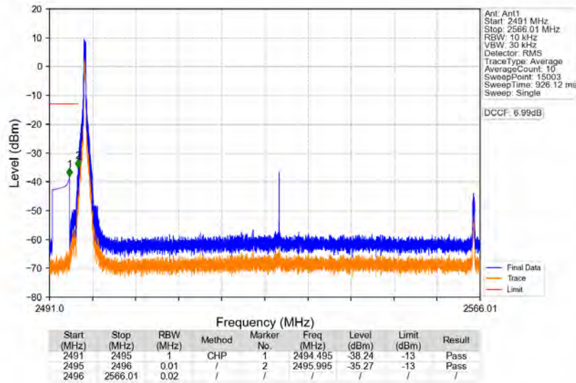
n41_30kHz_SISO_NTNV_70MHz_CP-OFDM_QPSK_2531.01MHz_Edge_1RB_Left
