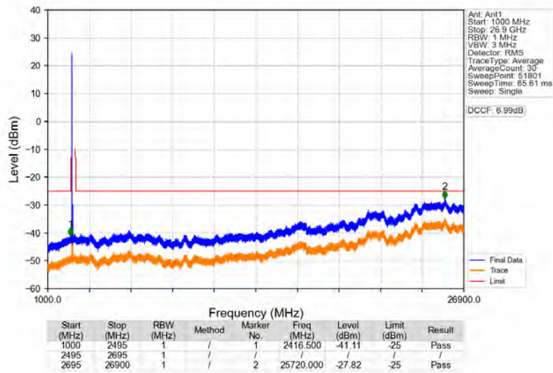
n41_30kHz_SISO_NTNV_60MHz_DFT-s-OFDM_PI/2_BPSK_2526MHz_Edge_1RB_Left
