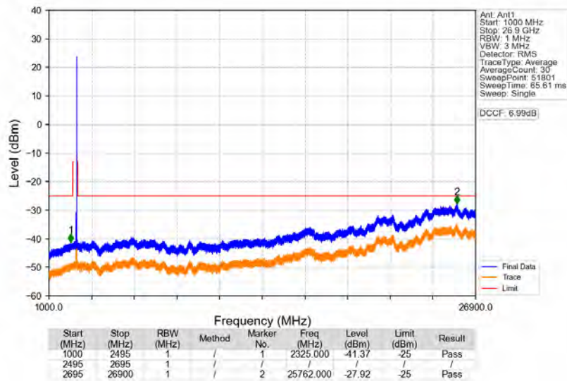
n41_30kHz_SISO_NTNV_60MHz_DFT-s-OFDM_PI/2_BPSK_2659.98MHz_Edge_1RB_Right
