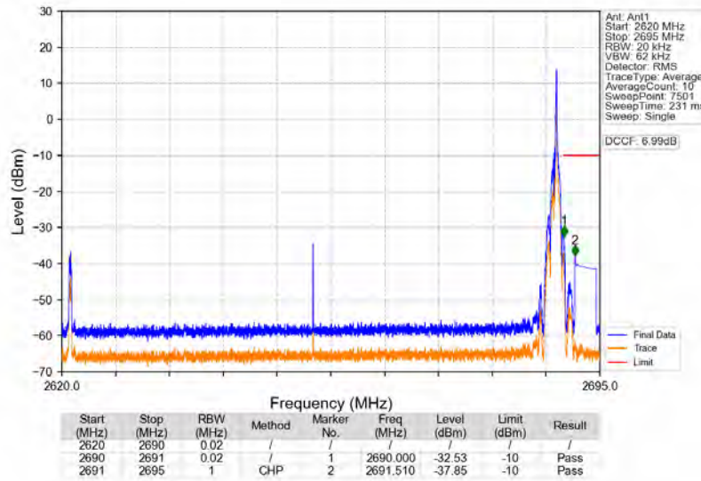
n41_30kHz_SISO_NTNV_70MHz_DFT-s-OFDM_PI/2_BPSK_2655MHz_Edge_1RB_Right
