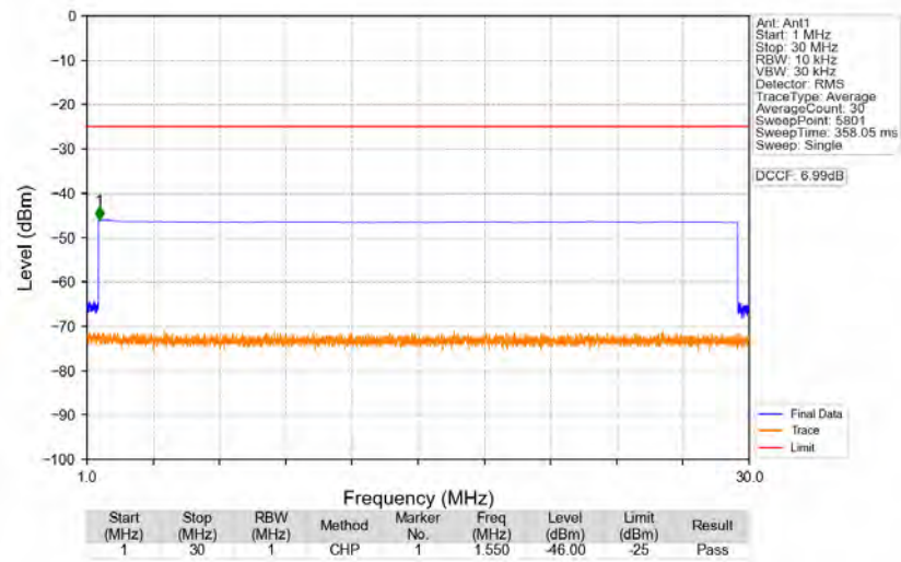
n41_30kHz_SISO_NTNV_70MHz_CP-OFDM_QPSK_2655MHz_Edge_1RB_Right
