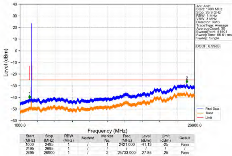
n41_30kHz_SISO_NTNV_70MHz_DFT-s-OFDM_PI/2_BPSK_2655MHz_Edge_1RB_Right
