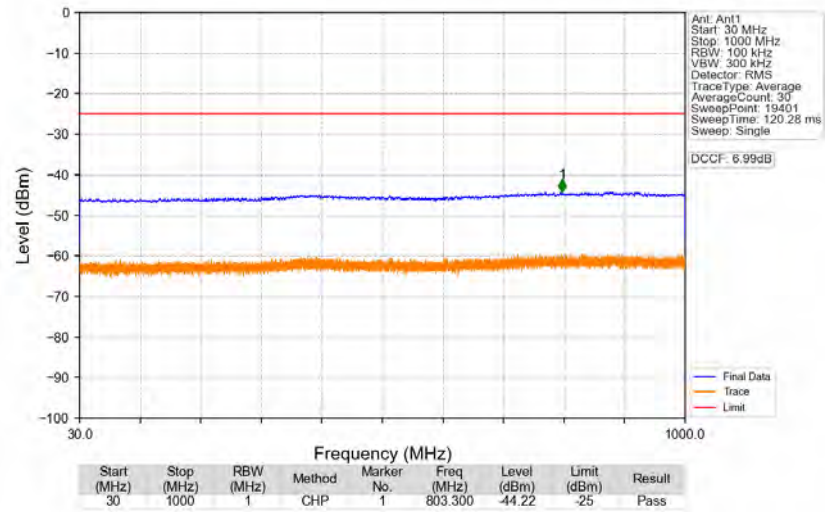
n41_30kHz_SISO_NTNV_70MHz_DFT-s-OFDM_QPSK_2655MHz_Edge_1RB_Right
