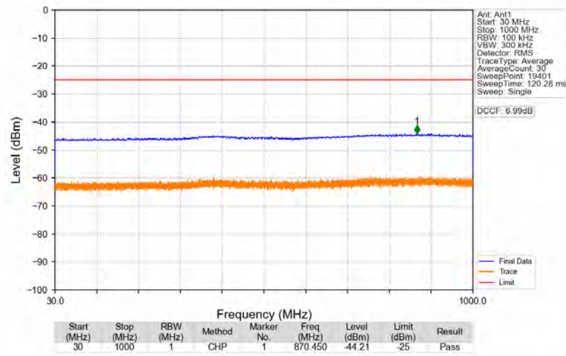
n41_30kHz_SISO_NTNV_60MHz_CP-OFDM_QPSK_2592.99MHz_Edge_1RB_Left
