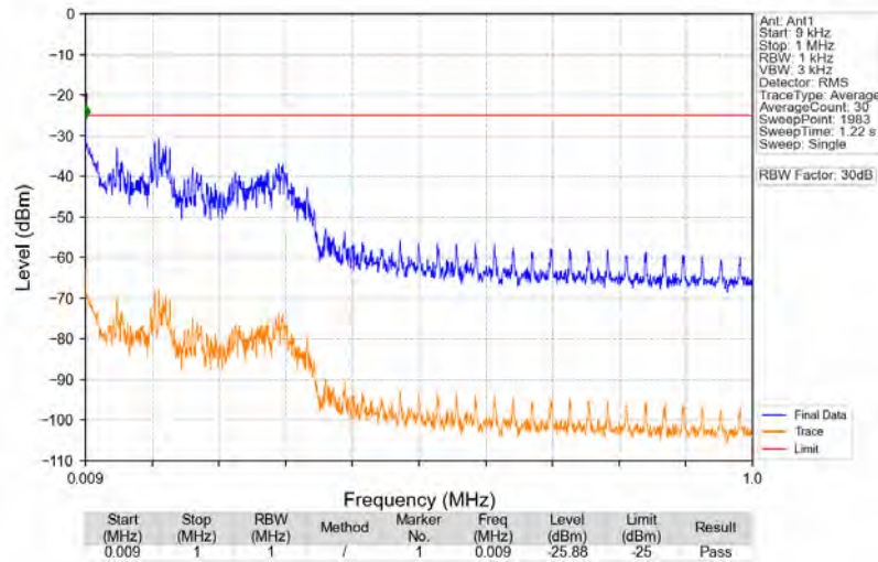
n41_30kHz_SISO_NTNV_70MHz_DFT-s-OFDM_PI/2_BPSK_2655MHz_Edge_1RB_Right
