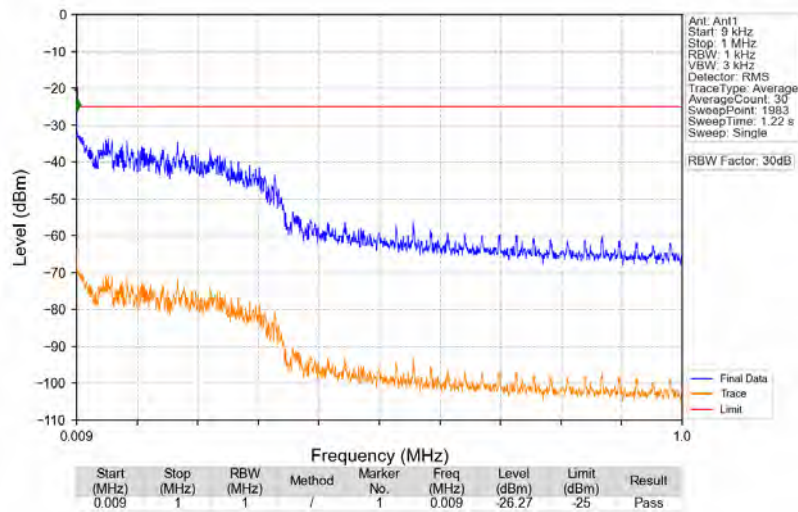
n41_30kHz_SISO_NTNV_70MHz_CP-OFDM_QPSK_2655MHz_Edge_1RB_Right
