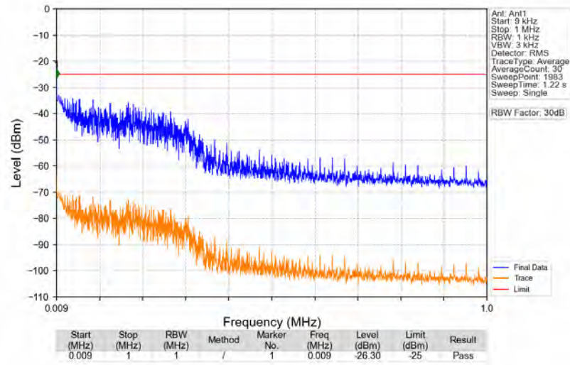
n41_30kHz_SISO_NTNV_60MHz_CP-OFDM_QPSK_2592.99MHz_Edge_1RB_Left
