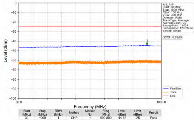
n41_30kHz_SISO_NTNV_70MHz_CP-OFDM_QPSK_2531.01MHz_Edge_1RB_Left
