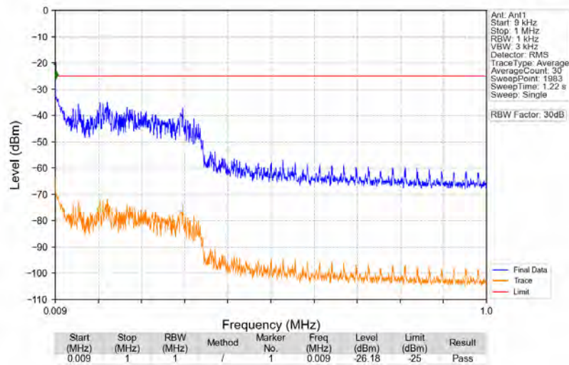
n41_30kHz_SISO_NTNV_70MHz_DFT-s-OFDM_QPSK_2655MHz_Edge_1RB_Right
