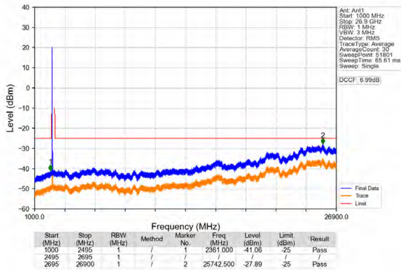
n41_30kHz_SISO_NTNV_60MHz_DFT-s-OFDM_QPSK_2526MHz_Edge_1RB_Left
