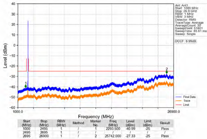
n41_30kHz_SISO_NTNV_70MHz_CP-OFDM_QPSK_2655MHz_Edge_1RB_Right
