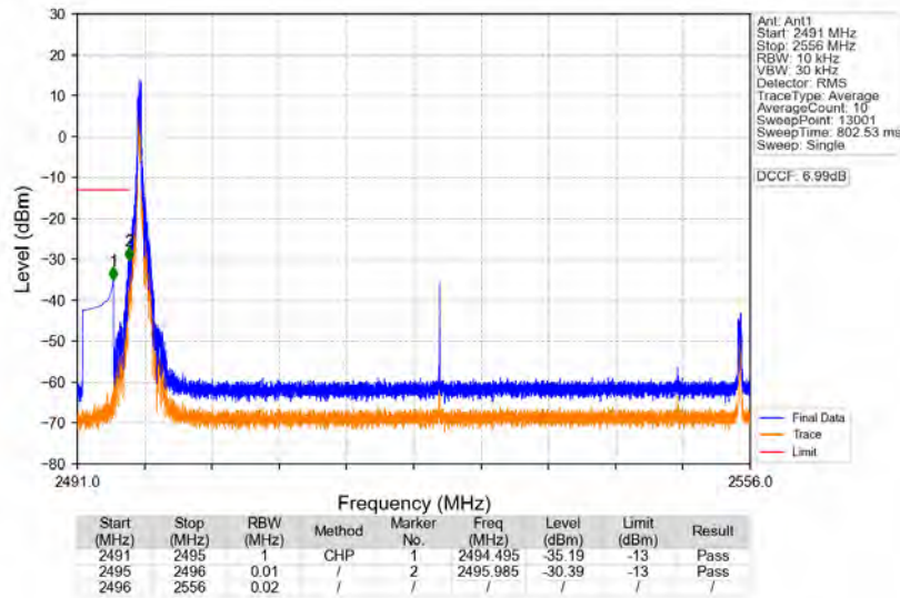
n41_30kHz_SISO_NTNV_60MHz_DFT-s-OFDM_QPSK_2526MHz_Edge_1RB_Left
