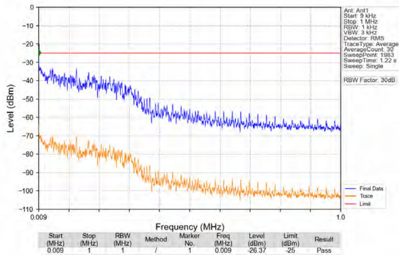
n41_30kHz_SISO_NTNV_60MHz_CP-OFDM_QPSK_2526MHz_Edge_1RB_Left
