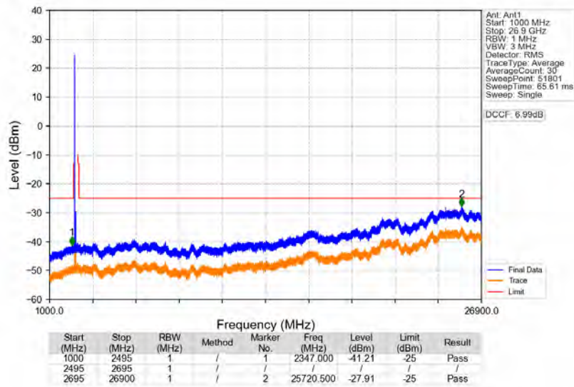
n41_30kHz_SISO_NTNV_70MHz_CP-OFDM_QPSK_2531.01MHz_Edge_1RB_Left
