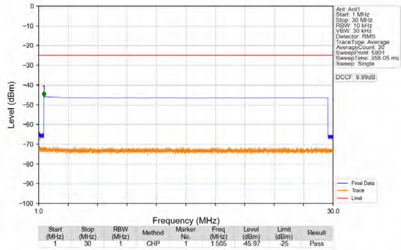
n41_30kHz_SISO_NTNV_70MHz_DFT-s-OFDM_QPSK_2655MHz_Edge_1RB_Right
