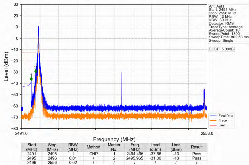
n41_30kHz_SISO_NTNV_60MHz_CP-OFDM_QPSK_2526MHz_Edge_1RB_Left
