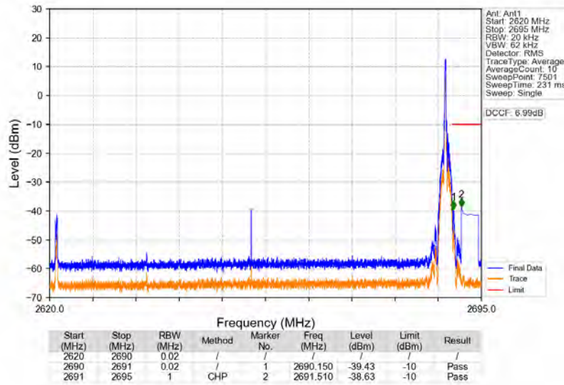
n41_30kHz_SISO_NTNV_70MHz_CP-OFDM_QPSK_2655MHz_Edge_1RB_Right
