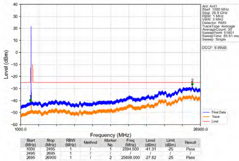
n41_30kHz_SISO_NTNV_60MHz_CP-OFDM_QPSK_2526MHz_Edge_1RB_Left
