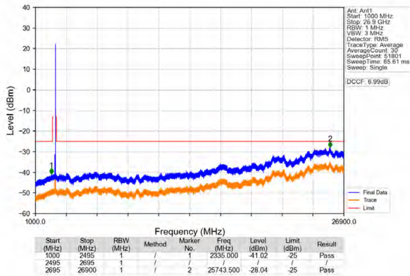
n41_30kHz_SISO_NTNV_70MHz_DFT-s-OFDM_QPSK_2655MHz_Edge_1RB_Right
