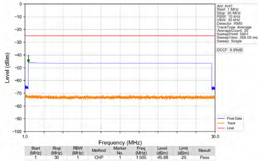
n41_30kHz_SISO_NTNV_60MHz_DFT-s-OFDM_QPSK_2526MHz_Edge_1RB_Left
