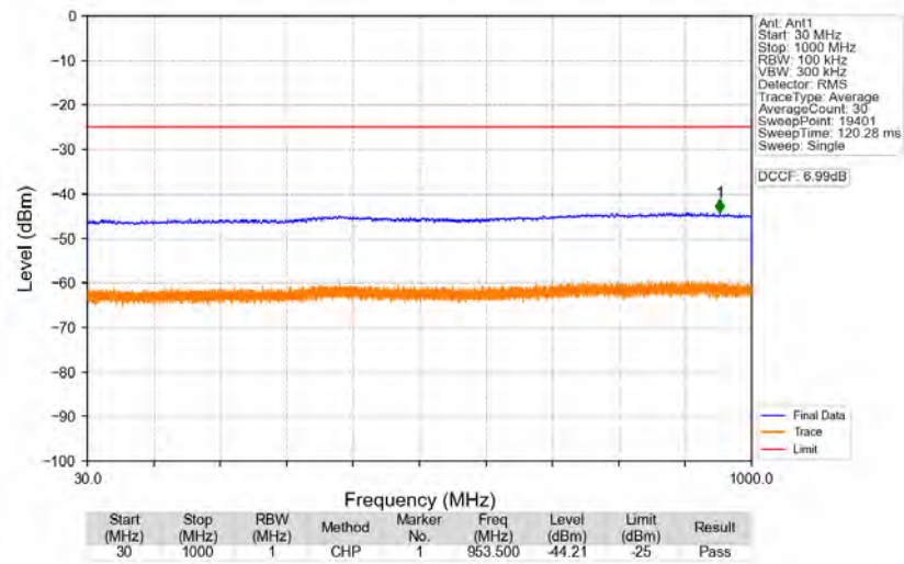
n41_30kHz_SISO_NTNV_60MHz_DFT-s-OFDM_PI/2_BPSK_2526MHz_Edge_1RB_Left
