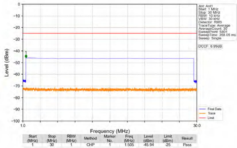
n41_30kHz_SISO_NTNV_60MHz_CP-OFDM_QPSK_2592.99MHz_Edge_1RB_Left
