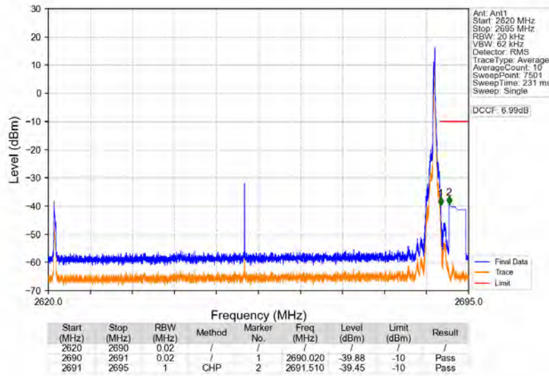
n41_30kHz_SISO_NTNV_70MHz_DFT-s-OFDM_QPSK_2655MHz_Edge_1RB_Right
