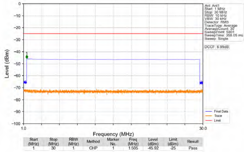
n41_30kHz_SISO_NTNV_70MHz_DFT-s-OFDM_PI/2_BPSK_2655MHz_Edge_1RB_Right
