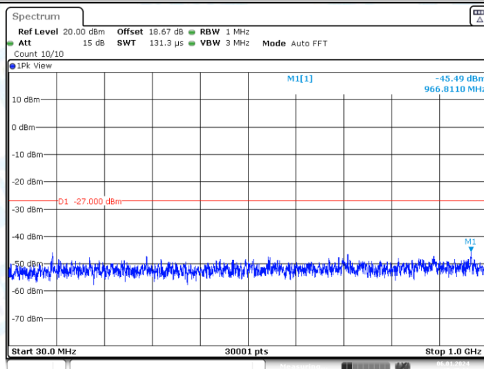
11N40-CDD_Ant2_5550_30~1000
