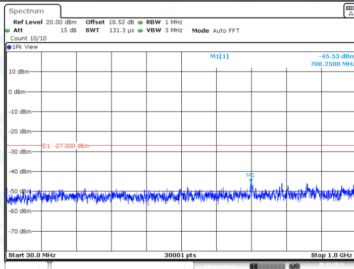
11AC20-CDD_Ant2_5280_30~1000
