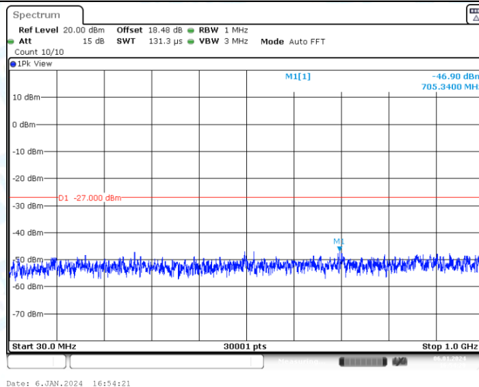
11AC20-CDD_Ant2_5200_1000~40000
