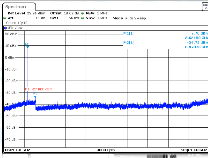
11N40-CDD_Ant1_5550_1000~40000
