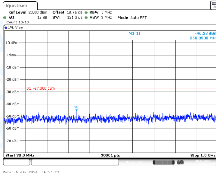
11N40-CDD_Ant1_5755_1000~40000
