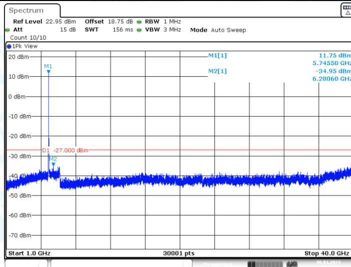
11AC20-CDD_Ant1_5745_1000~40000
