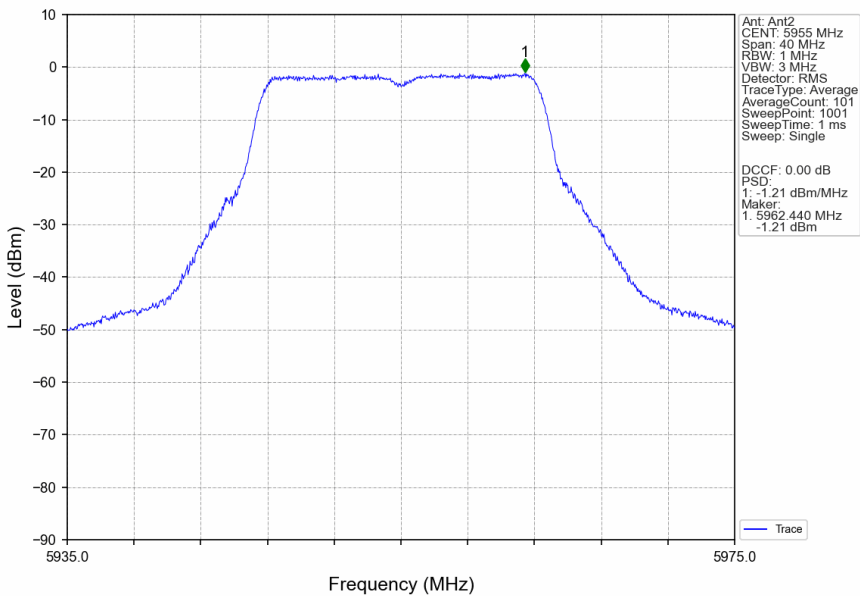
802.11a_LCH_5955MHz_Ant2_NTNV
