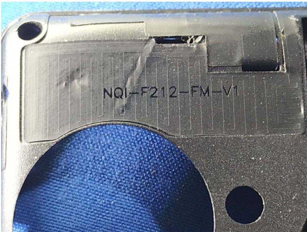
FM ANT
