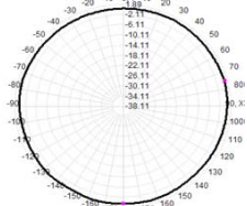
Total(H+V), Max= 0.86dB, CrD=1.30
