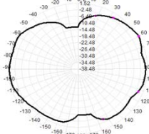
2490.0MHz Total(E2-YZ), Max= 1.89dB
