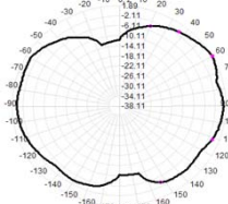
2500.0MHz Total(E2-YZ), Max= 1.89dB
