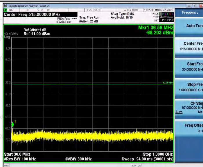
802.11n(HT20)SISO_Ant1_2462_30~1000
