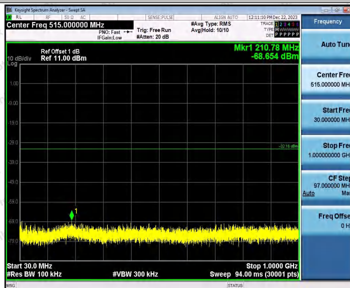
802.11n(HT40)SISO_Ant2_2437_30~1000
