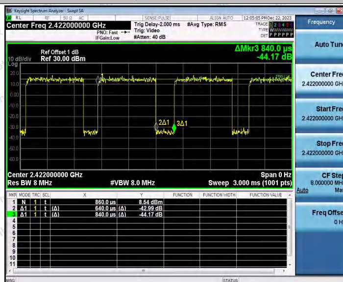
802.11n(HT40)SISO_Ant2_2422
