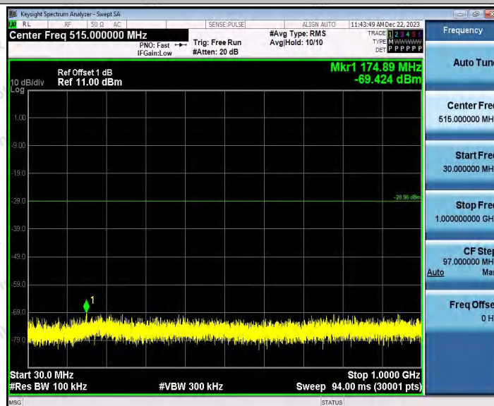
802.11g_Ant2_2462_30~1000
