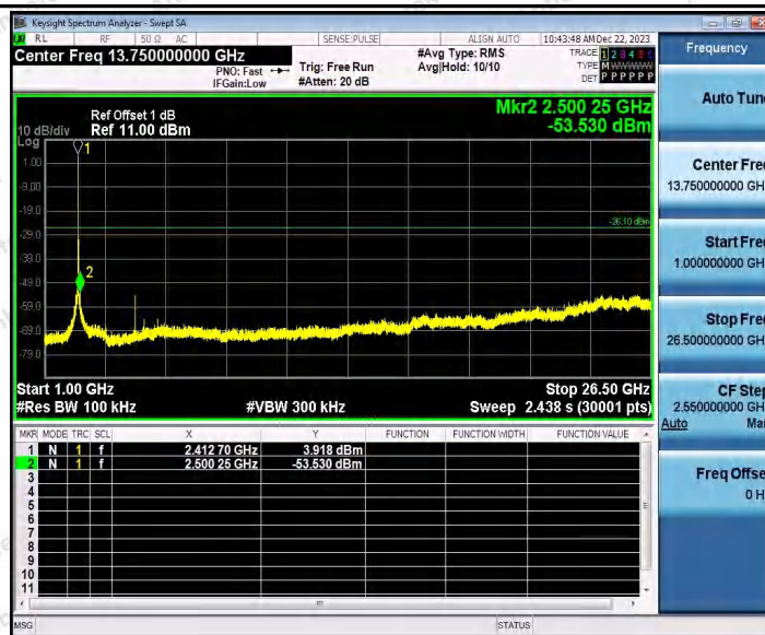
802.11b_Ant2_2412_0~Reference
