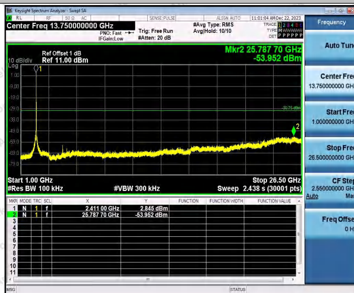
802.11n(HT20)SISO_Ant2_2412_0~Reference
