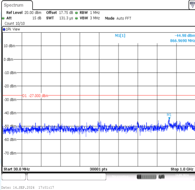
11N20MIMO-Ant1-5745-30~1000-PASS
