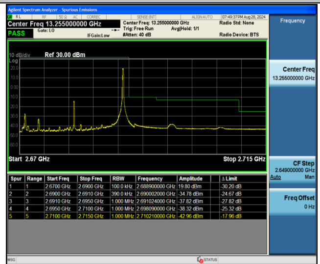
Band41-20MHz-QPSK-41490-1RB#99-PASS
