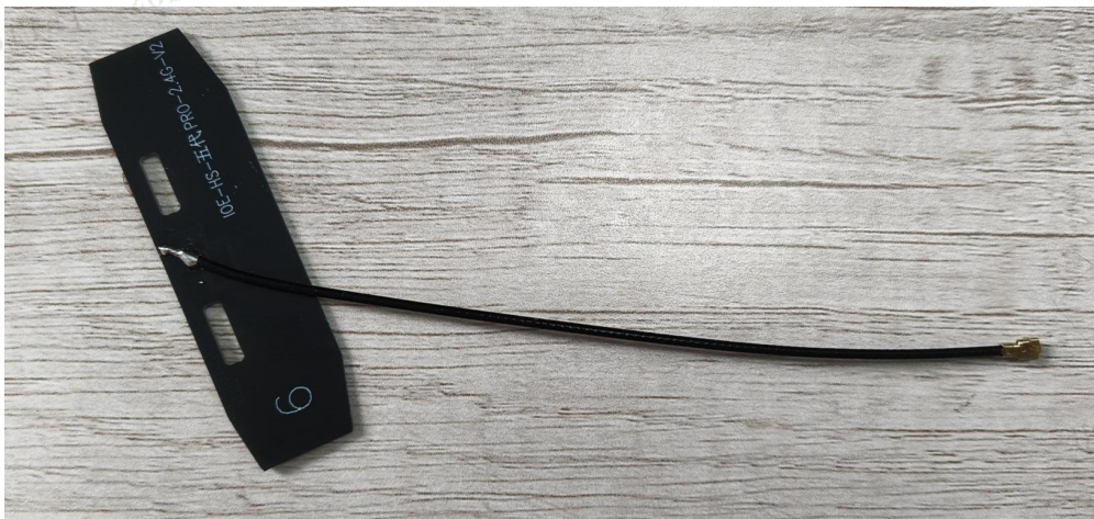
HS-五代 PRO-6#-2.4G 全向天线 PCB 黑色 To IPEX 一代 OD1.37mm 黑色低损线 L120mm
