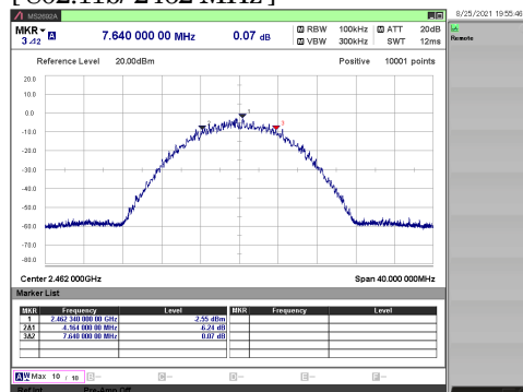
[ 802.11b/ 2462 MHz ]
