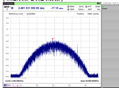
[ 802.11b/ 2462 MHz ]
