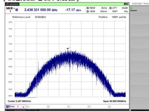
[ 802.11b/ 2437 MHz ]
