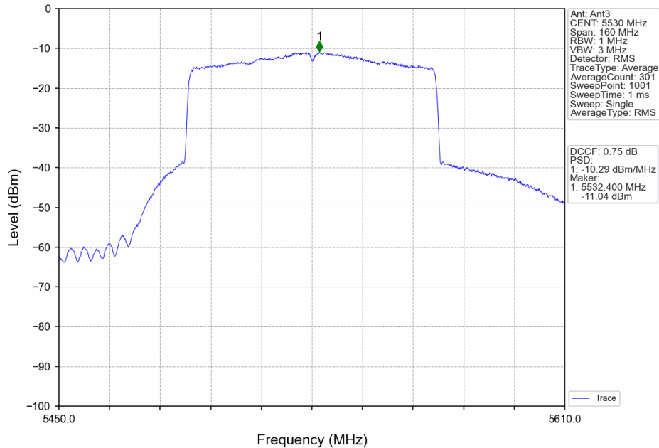
802.11ax(HEW80)_LCH_5530MHz_RU996_Left_MIMO_NTNV
