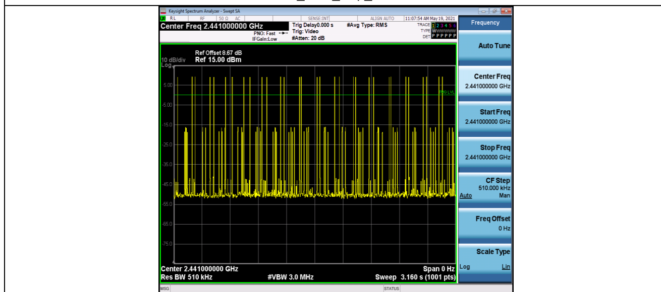
DH1_Ant1_Hop_2441
