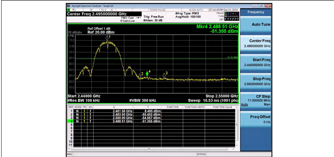
802.11b-Ant1-2462-PASS
