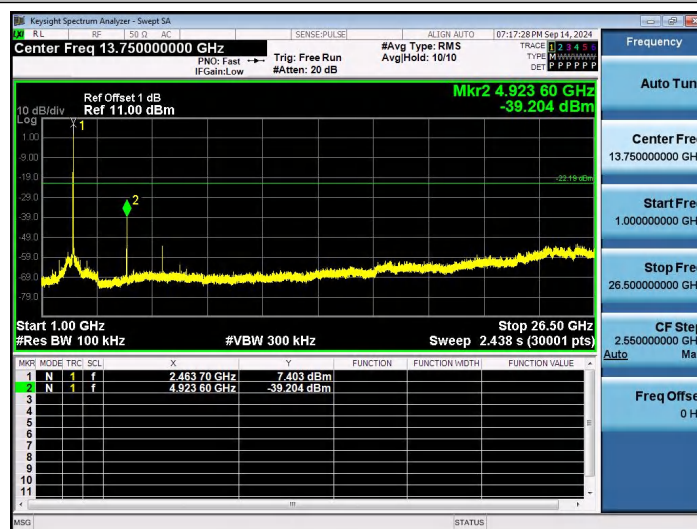
802.11b-Ant1-2462-1000~26500-PASS
