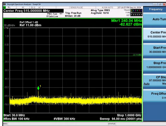
802.11b-Ant1-2462-30~1000-PASS
