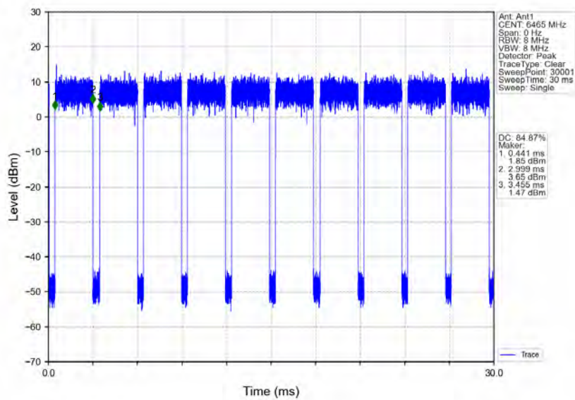
802.11ax(HEW80)_LCH_6465MHz_RU996_Left_Ant1_NTNV
