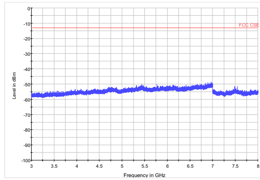
LTE Band 135MHz CH-Middle 3GHz~8GHz
