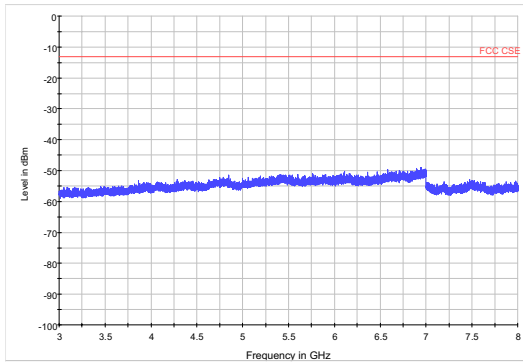
LTE Band 1210MHzCH-Middle 3GHz~8GHz
