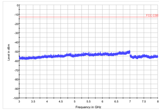
LTE Band 1310MHz CH-Middle 3GHz~8GHz
