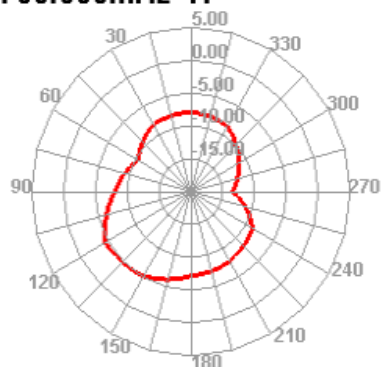
700.000MHz H
