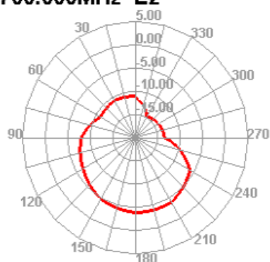
700.000MHz E2
