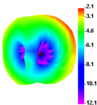
900.000MHz
