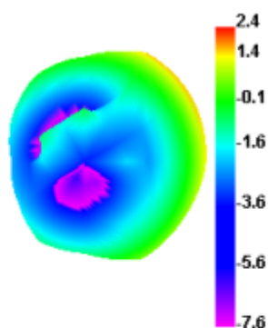
3300.000MHz E1
