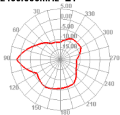
2400.000MHz E1
