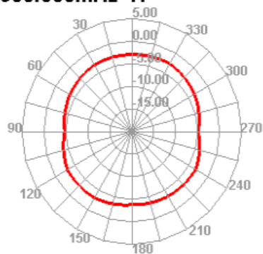
900.000MHz H
