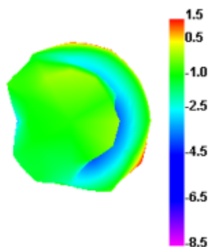
4200.000MHz E1
