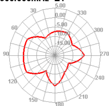
900.000MHz E1
