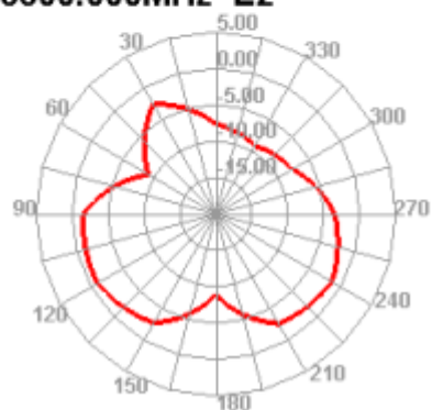
3300.000MHz E2
