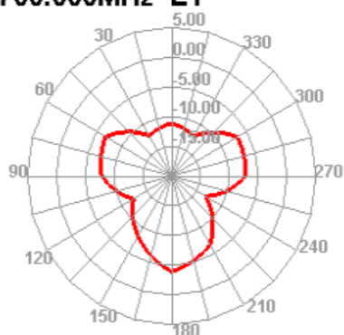
700.000MHz E1
