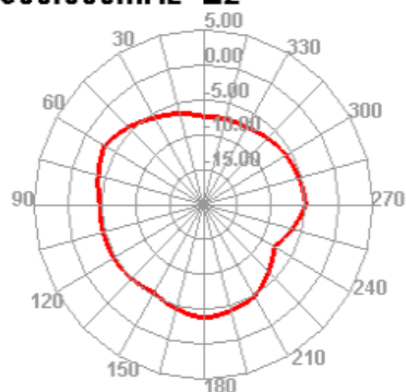
900.000MHz E2
