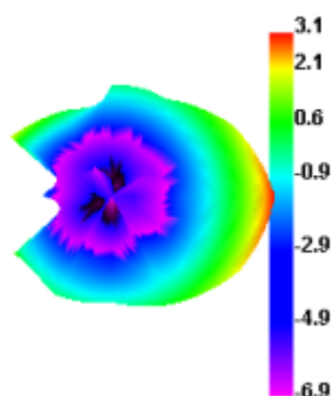
2700.000MHz E1
