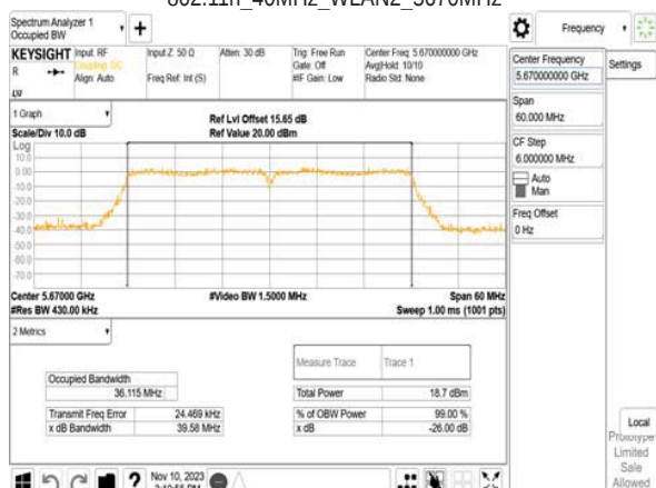
802.11n_40MHz_WLAN2_5670MHz
