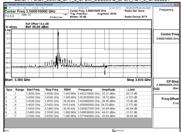
Band77-Part27 90MHz DFT_s OFDM_SCS30kHz BPSK RB1_0 CH633334
