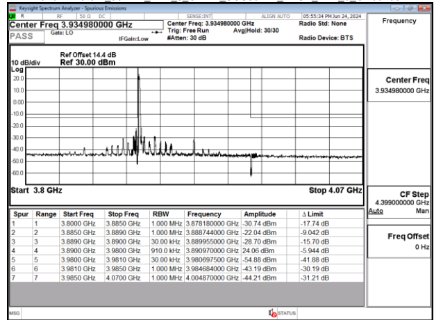
Band77-Part27_90MHz_DFT_s_OFDM_SCS30kHz_BPSK_RB1_244_CH633000
