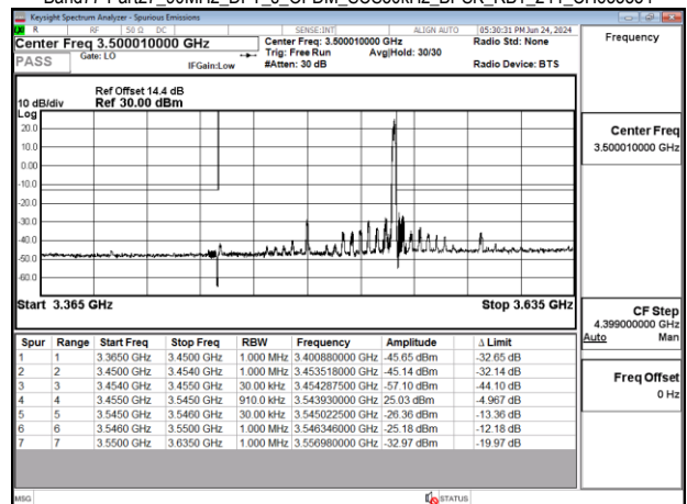
Band77-Part27_90MHz_DFT_s_OFDM_SCS30kHz_BPSK_RB1_244_CH633334
