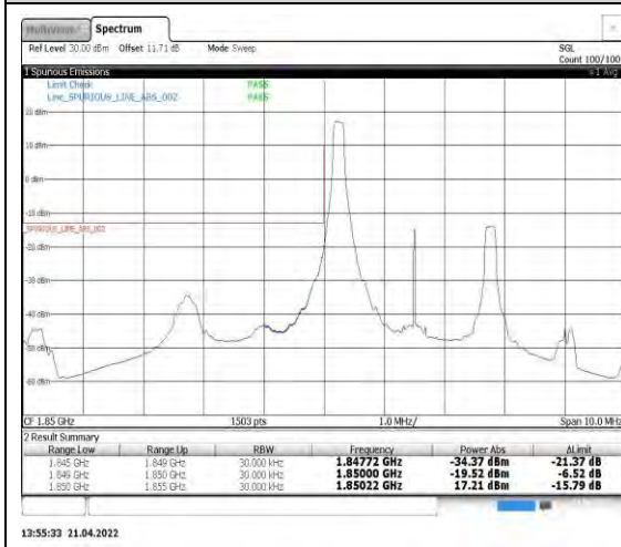
Band2-3MHz-QPSK-18615-1RB#0
