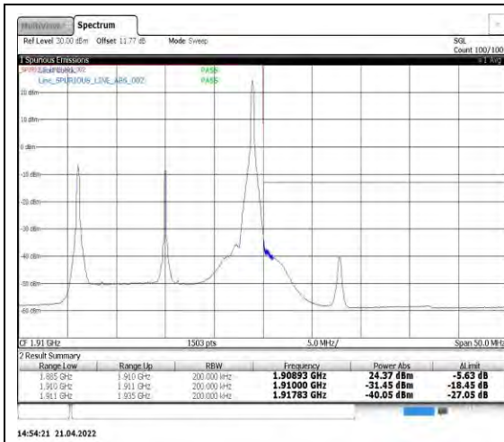
Band2-20MHz-QPSK-19100-1RB#99
