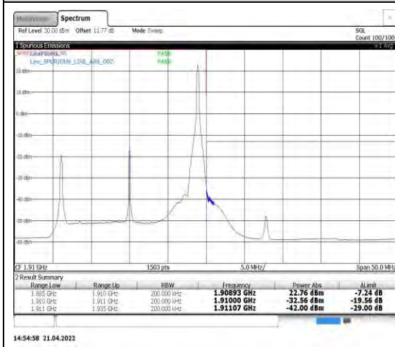
Band2-20MHz-16QAM-19100-1RB#99
