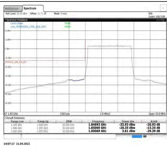
Band2-3MHz-16QAM-18615-15RB#0
