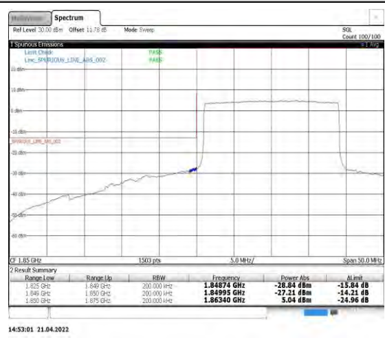
Band2-20MHz-QPSK-18700-100RB#0
