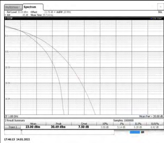
Band2-20MHz-16QAM-18900
