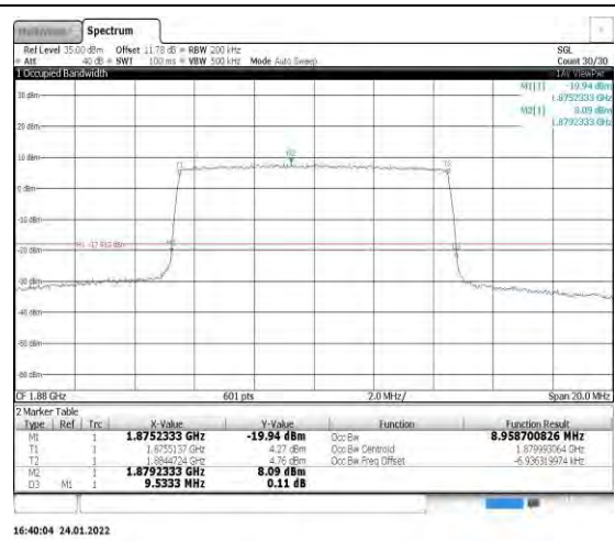
Band2-10MHz-16QAM-18900-50RB#0
