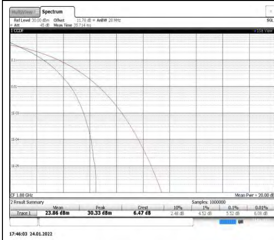
Band2-20MHz-QPSK-18900
