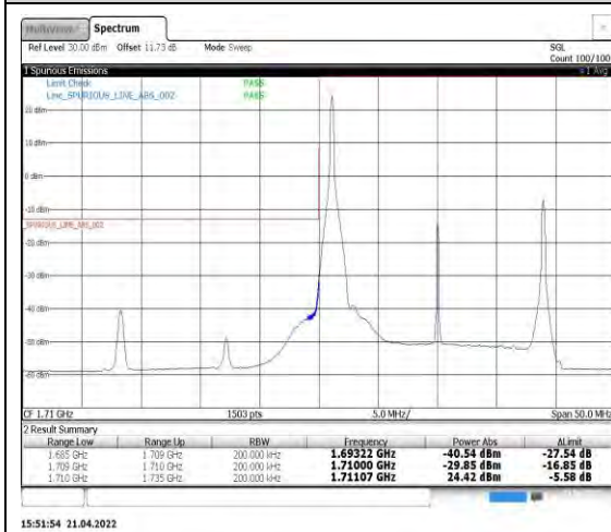
Band4-20MHz-QPSK-20050-1RB#0
