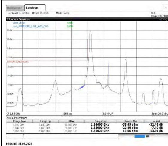
Band2-5MHz-QPSK-18625-1RB#0
