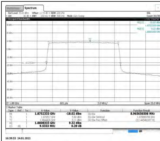
Band2-10MHz-QPSK-18900-50RB#0
