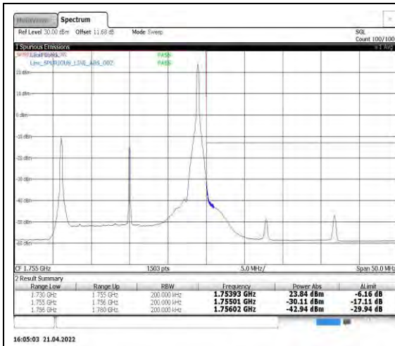
Band4-20MHz-QPSK-20300-1RB#99
