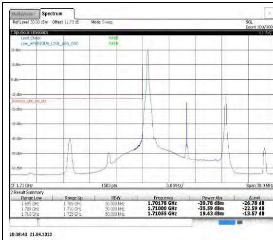
Band4-10MHz-QPSK-20000-1RB#0
