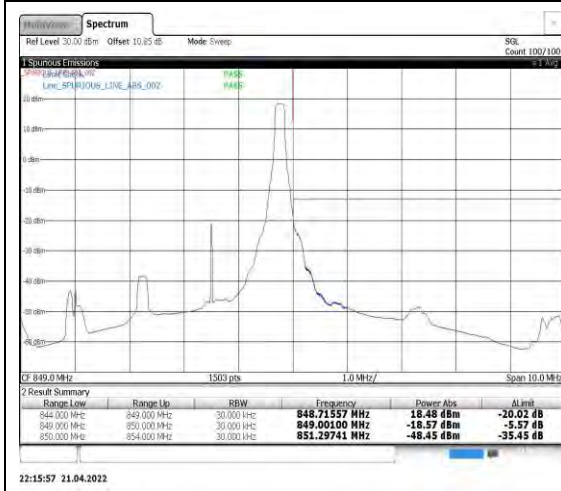
Band5-3MHz-QPSK-20635-1RB#14
