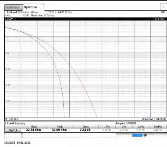
Band2-15MHz-16QAM-18900
