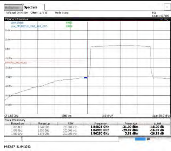
Band2-20MHz-16QAM-18700-100RB#0
