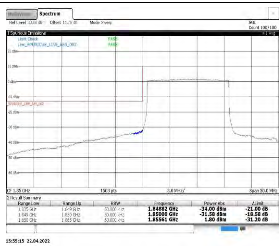
Band2-10MHz-QPSK-18650-50RB#0
