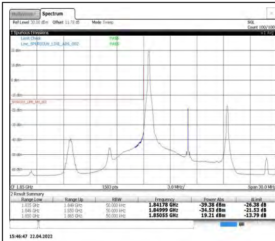
Band2-10MHz-QPSK-18650-1RB#0
