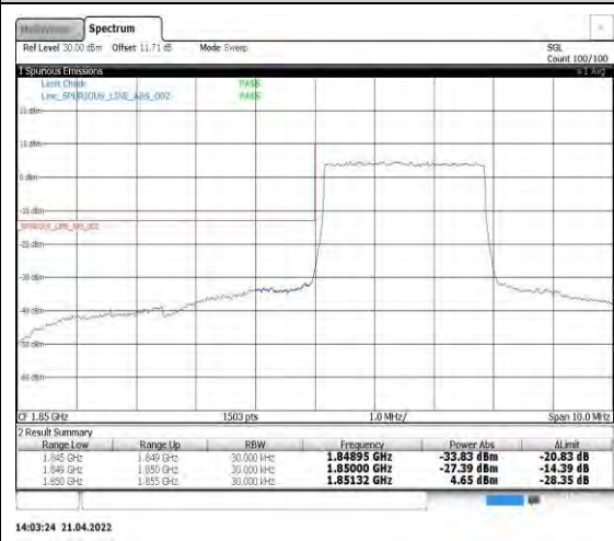
Band2-3MHz-QPSK-18615-15RB#0
