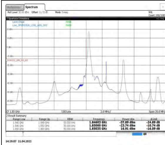
Band2-5MHz-16QAM-18625-1RB#0
