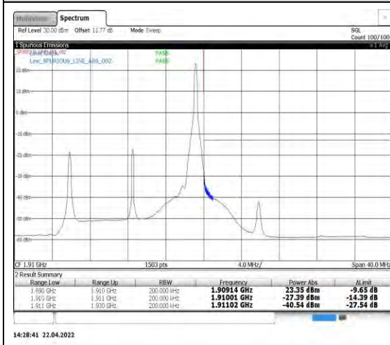
Band2-15MHz-16QAM-19125-1RB#74
