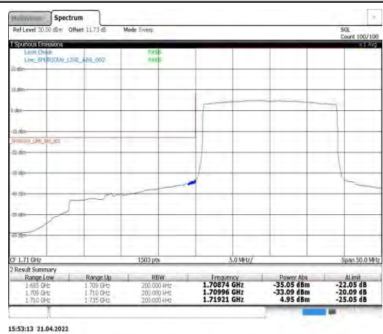
Band4-20MHz-QPSK-20050-100RB#0
