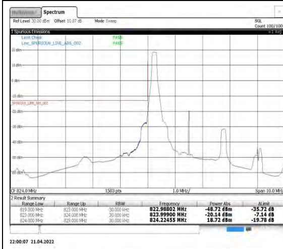
Band5-3MHz-QPSK-20415-1RB#0
