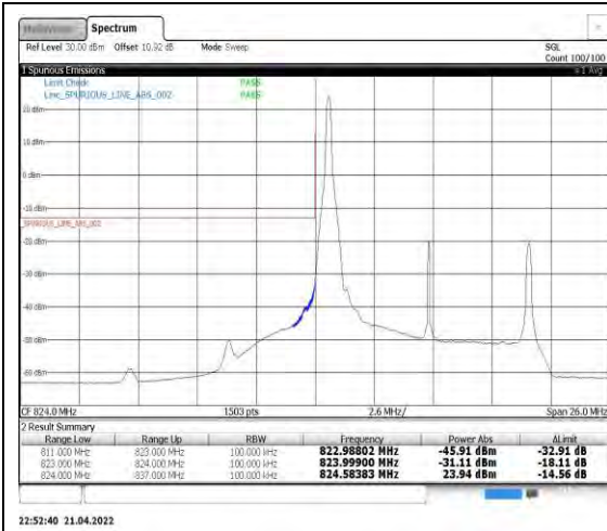
Band5-10MHz-QPSK-20450-1RB#0
