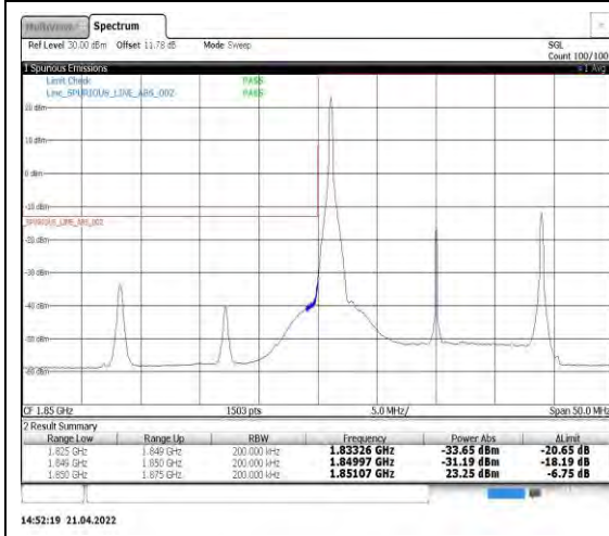
Band2-20MHz-16QAM-18700-1RB#0
