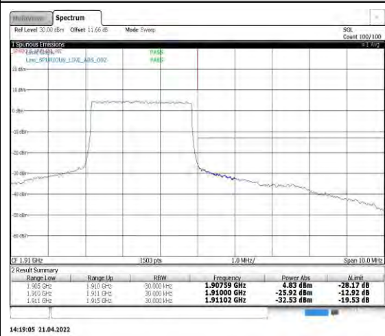
Band2-3MHz-QPSK-19185-15RB#0
