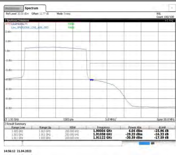
Band2-20MHz-16QAM-19100-100RB#0
