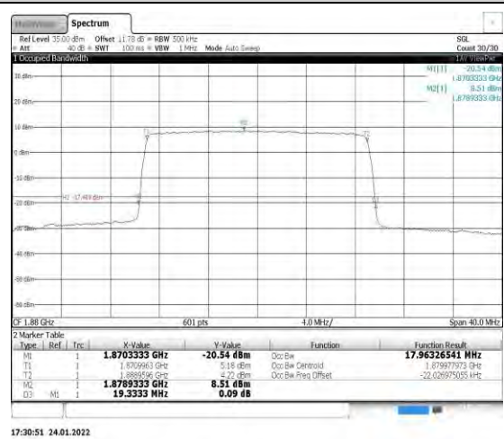
Band2-20MHz-16QAM-18900-100RB#0
