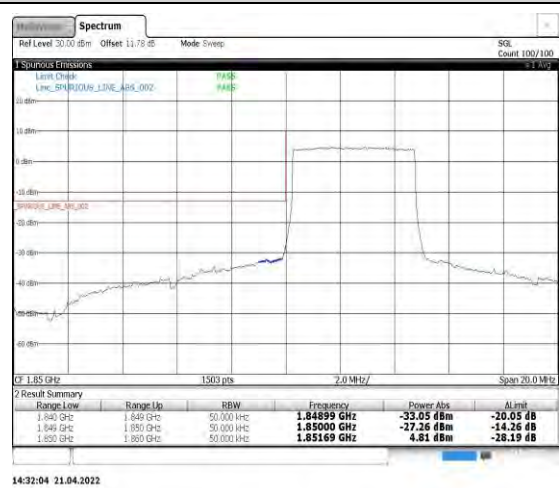
Band2-5MHz-QPSK-18625-25RB#0
