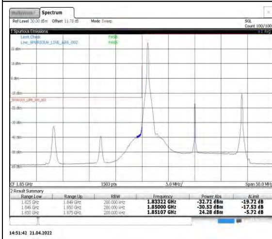
Band2-20MHz-QPSK-18700-1RB#0
