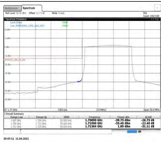
Band4-10MHz-QPSK-20000-50RB#0
