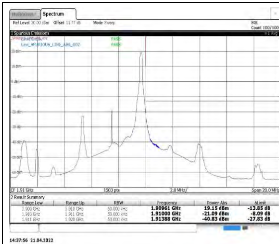
Band2-5MHz-QPSK-19175-1RB#24
