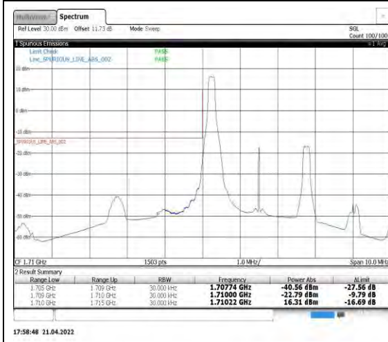
Band4-3MHz-QPSK-19965-1RB#0
