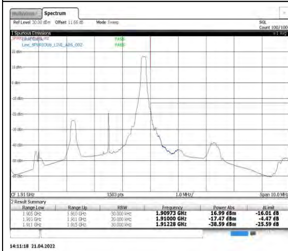
Band2-3MHz-QPSK-19185-1RB#14
