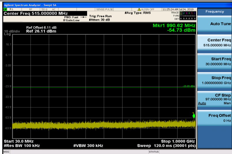
Band7-10MHz-QPSK-20800-1RB#0-30~1000MHz
