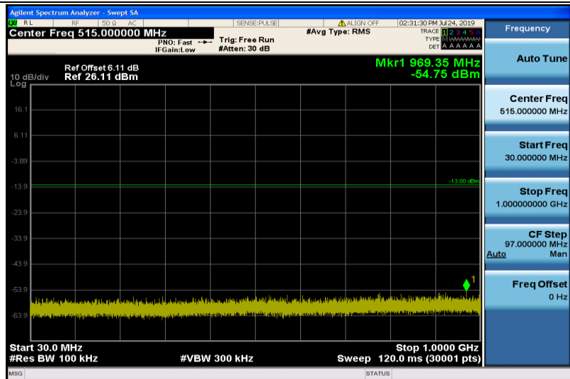
Band4-20MHz-QPSK-20050-1RB#0-30~1000MHz
