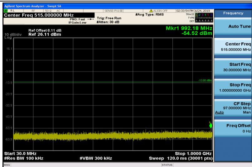
Band4-20MHz-QPSK-20300-1RB#0-30~1000MHz
