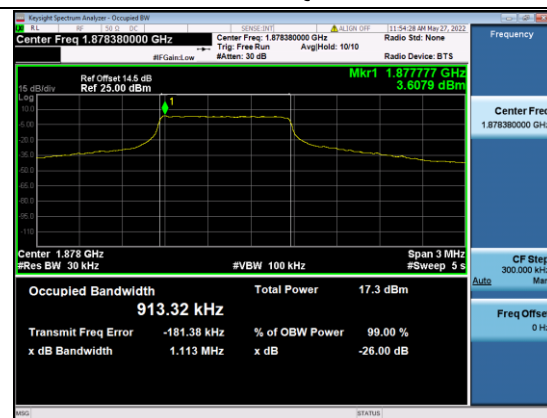
B2-5M-Mid CH-OBW-Q16
