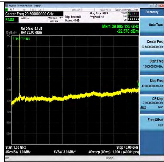
NTN-N78-3450-3550-PC2-30-60-L-CP-QPSK-Edge_1RB_L eft-Ant3-PASS
