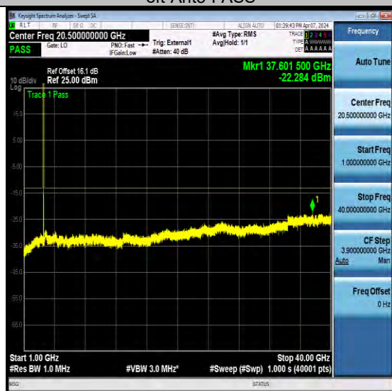
NTNV-N78-3450-3550-PC2-30-20-M-CP-QPSK-Edge_1RB_L Left-Ant5-PASS
