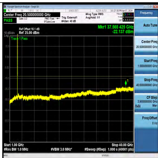
NTNV-N78-3450-3550-PC2-30-20-L-CP-QPSK-Edge_1RB_L eft-Ant5-PASS
