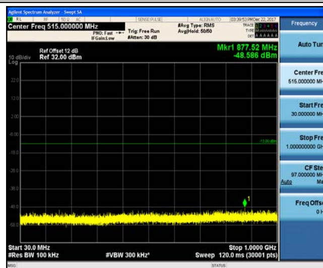
Band2 10MHz QPSK 18900 1RB#0
