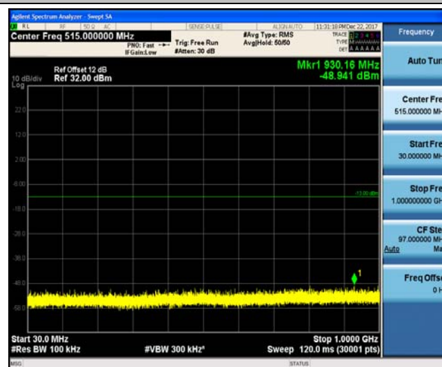
Band4 20MHz 16QAM 20175 1RB#0
