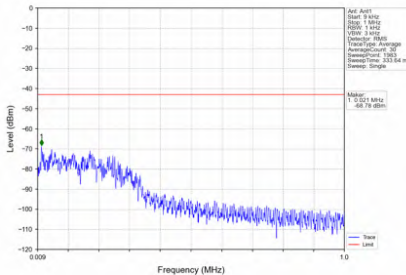
n7 30kHz SISO NTNv 30MHz CP-OFDM QPSK 2515MHz Edge 1RB Left
