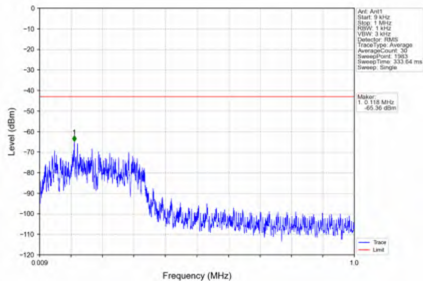
n7 30kHz SISO NTNv 20MHz DFT-s-OFDM QPSK 2560MHz Edge 1RB Right
