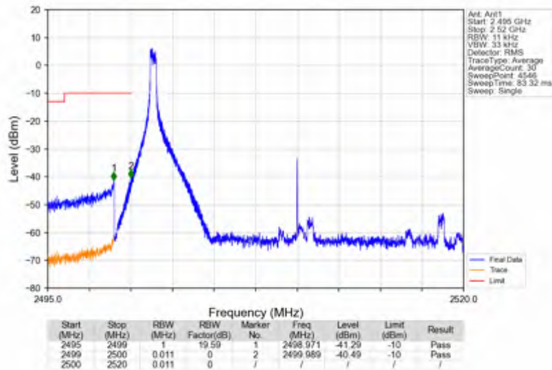
n7_30kHz_SISO_NTNV_20MHz_DFT-s-OFDM_QPSK_2510MHz_Inner_1RB_Left
