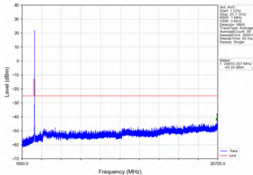
n7 30kHz SISO NTN 40MHz DFT-s-OFDM QPSK 2550MHz Edge 1RB Right
