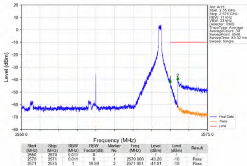
n7_30kHz_SISO_NTNV_20MHz_CP-OFDM QPSK_2560MHz_Inner_1RB_Right
