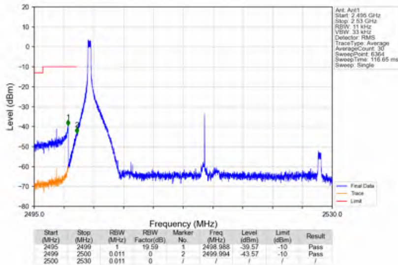
n7 30kHz SISO NTNv 30MHz CP-OFDM QPSK 2515MHz Inner 1RB Left
