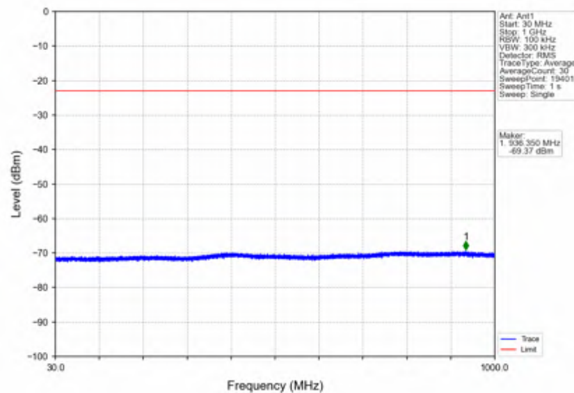
n7_15kHz_SISO_NTNV_50MHz_CP-OFDM QPSK_2525MHz_Inner_1RB_Left
