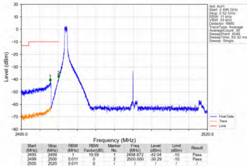
n7 30kHz SISO NTNv 20MHz CP-OFDM QPSK 2510MHz Edge 1RB Left
