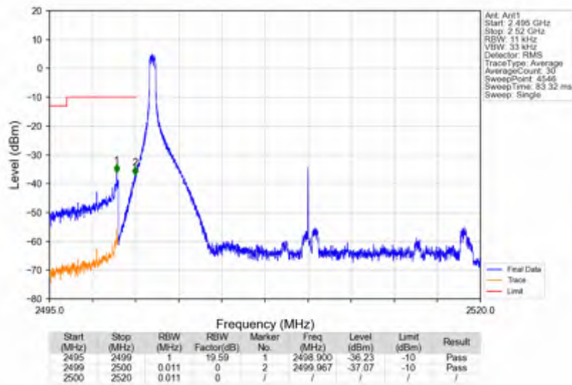
n7_30kHz_SISO_NTNV_20MHz_DFT-s-OFDM_PI/2_BPSK_2510MHz_Edge_1RB_Left
