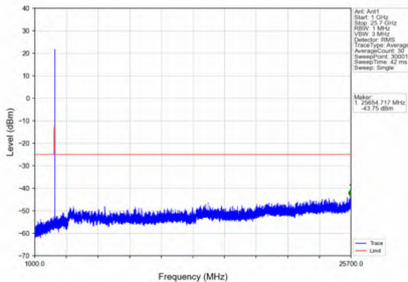
n7 30kHz SISO NTN 10MHz DFT-s-OFDM QPSK 2565MHz Edge 1RB Right
