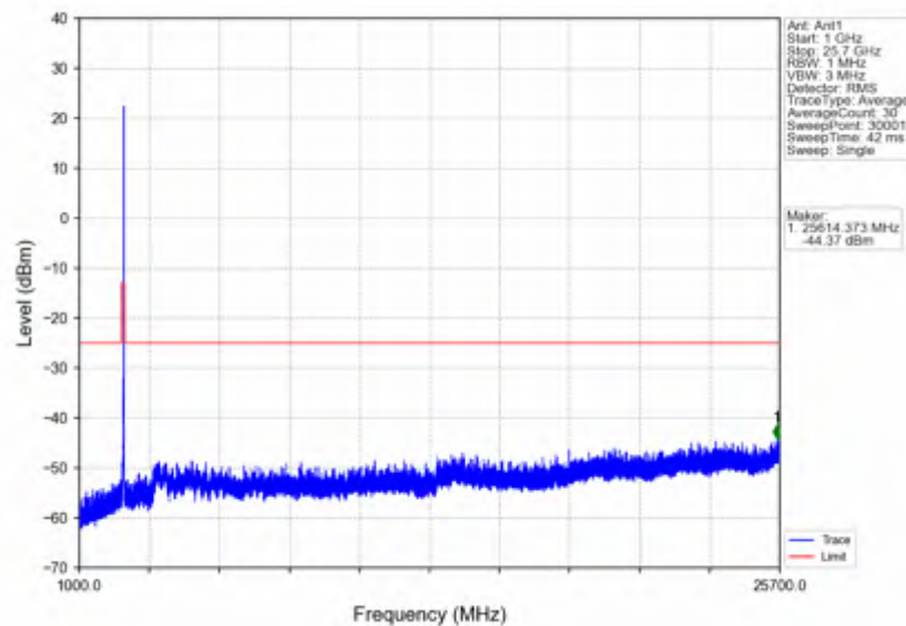
n7 30kHz SISO NTNV 25MHz DFT-s-OFDM PI/2 BPSK 2557.5MHz Edge 1RB Right
