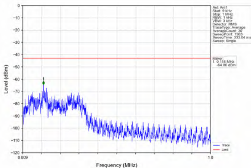
n7_30kHz_SISO_NTNV_20MHz_DFT-s-OFDM_PI/2_BPSK_2510MHz_Edge_1RB_Left
