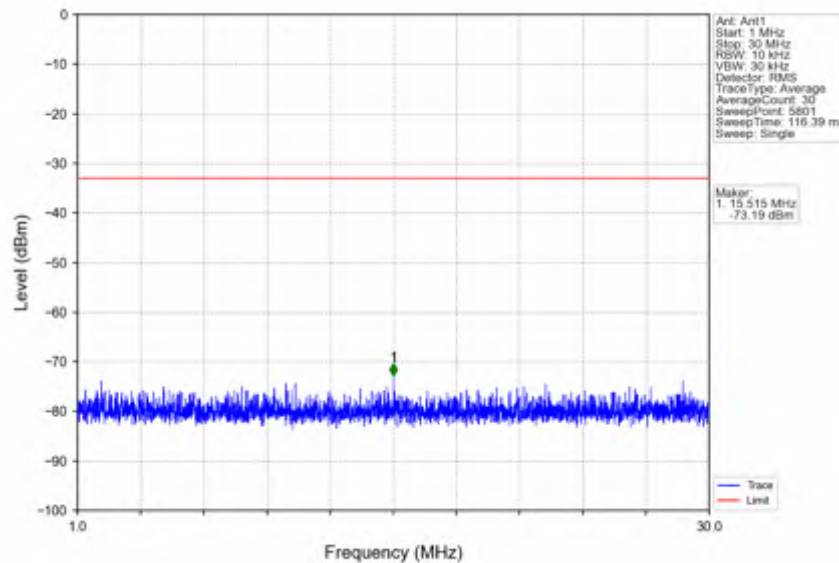
n7_30kHz_SISO_NTNV_20MHz_CP-OFDM QPSK_2510MHz_Edge_1RB_Left
