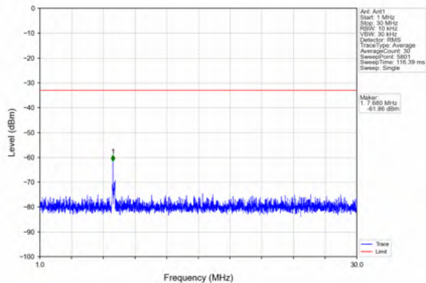
n7 30kHz SISO NTNv 25MHz DFT-s-OFDM PI/2 BPSK 2557.5MHz Edge 1RB Right
