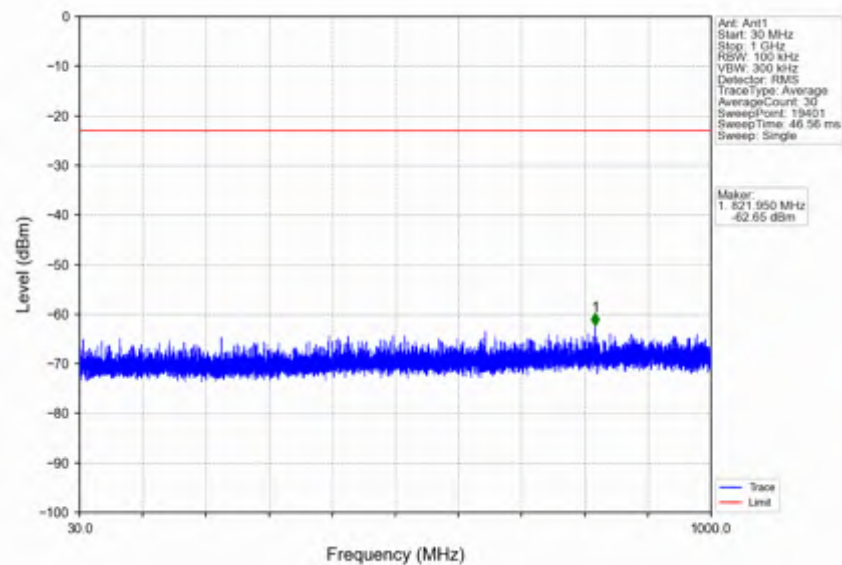
n7 30kHz SISO NTN 30MHz DFT-s-OFDM QPSK 2555MHz Edge 1RB Right
