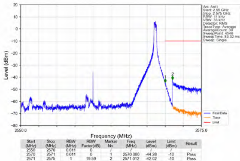
n7_30kHz_SISO_NTNV_20MHz_DFT-s-OFDM PI/2 BPSK_2560MHz_Inner_1RB_Right
