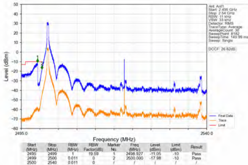
n7_30kHz_SISO_NTNV_40MHz_DFT-s-OFDM_QPSK_2520MHz_Inner_1RB_Left
