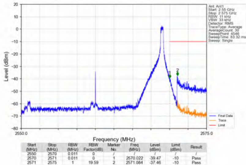
n7 30kHz SISO NTV 20MHz CP-OFDM QPSK 2560MHz Edge 1RB Right
