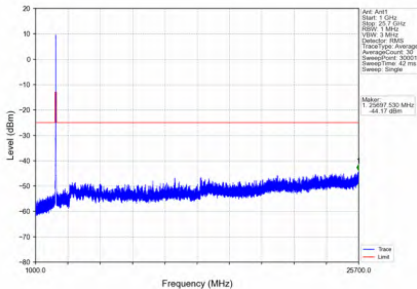
n7 30kHz SISO NTV 20MHz CP-OFDM QPSK 2560MHz Edge 1RB Right
