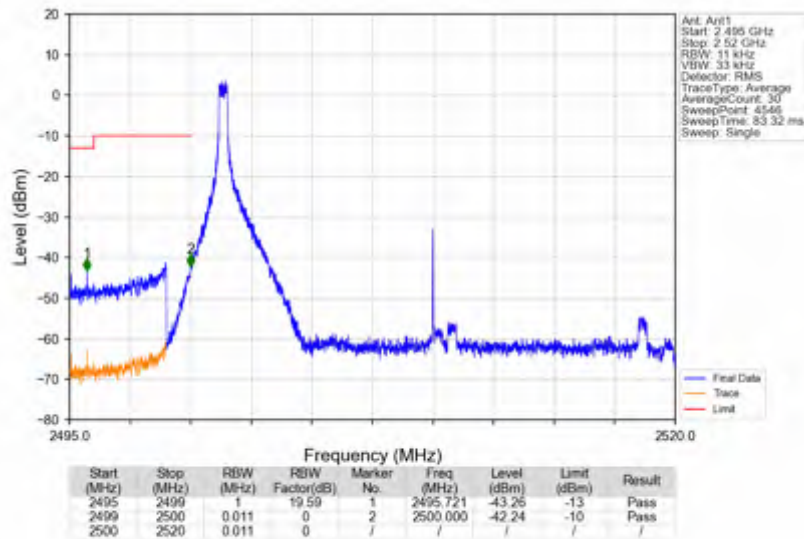
n7_30kHz_SISO_NTNV_20MHz_CP-OFDM QPSK_2510MHz_Inner_1RB_Left
