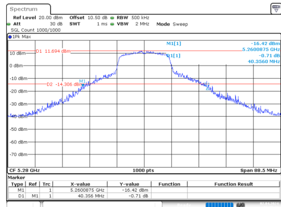
a_5280MHz_Chain 0
