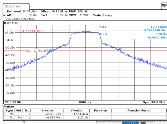
a_5320MHz_Chain 0
