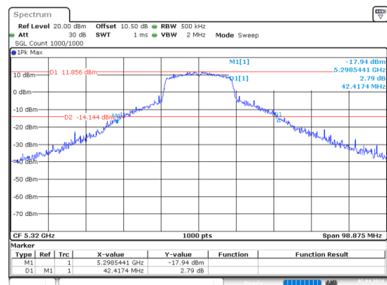
n20_5320MHz_Chain 0
