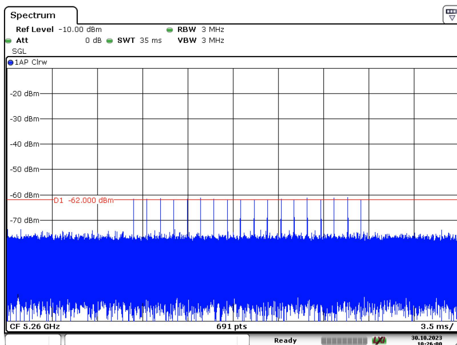
Radar Type 1A – 5260MHz
