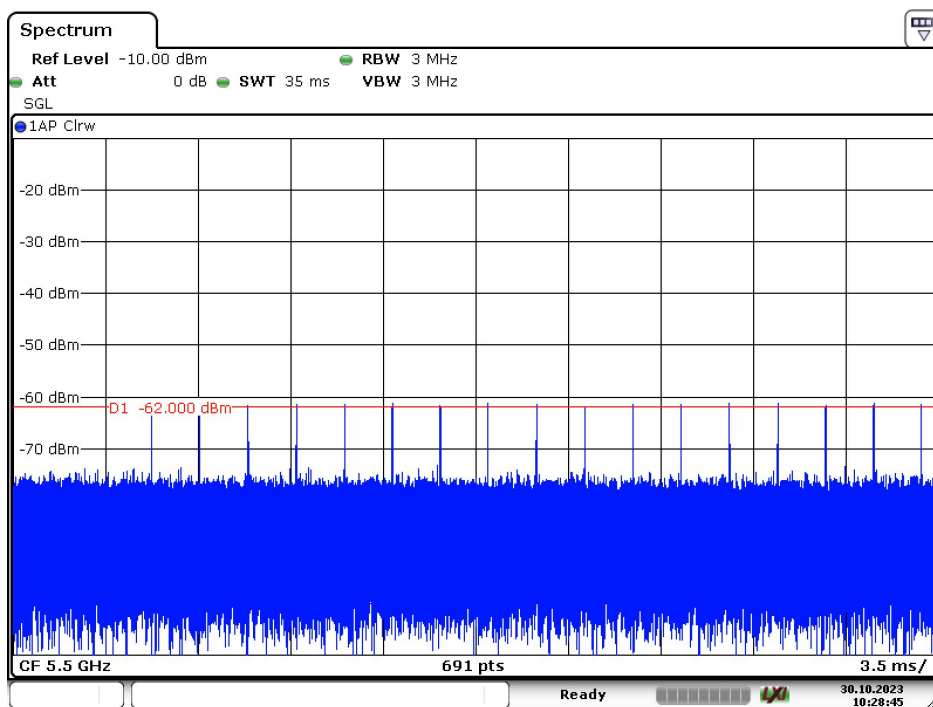
Radar Type 2 – 5500MHz
