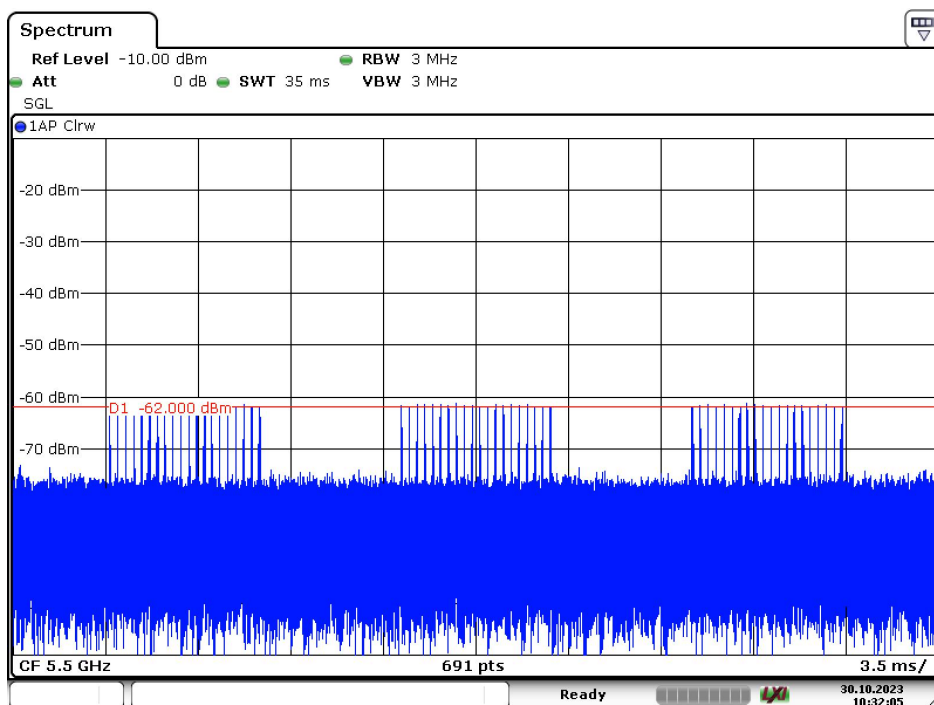
Radar Type 4 – 5500MHz
