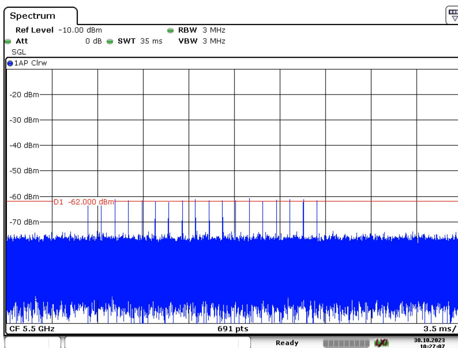
Radar Type 1A – 5500MHz
