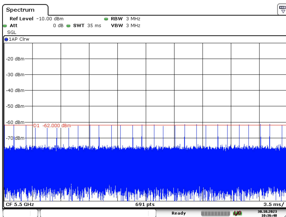
Radar Type 6 – 5500MHz
