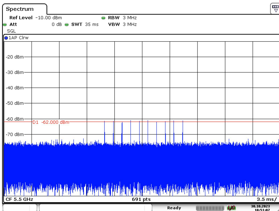
Radar Type 1B – 5500MHz
