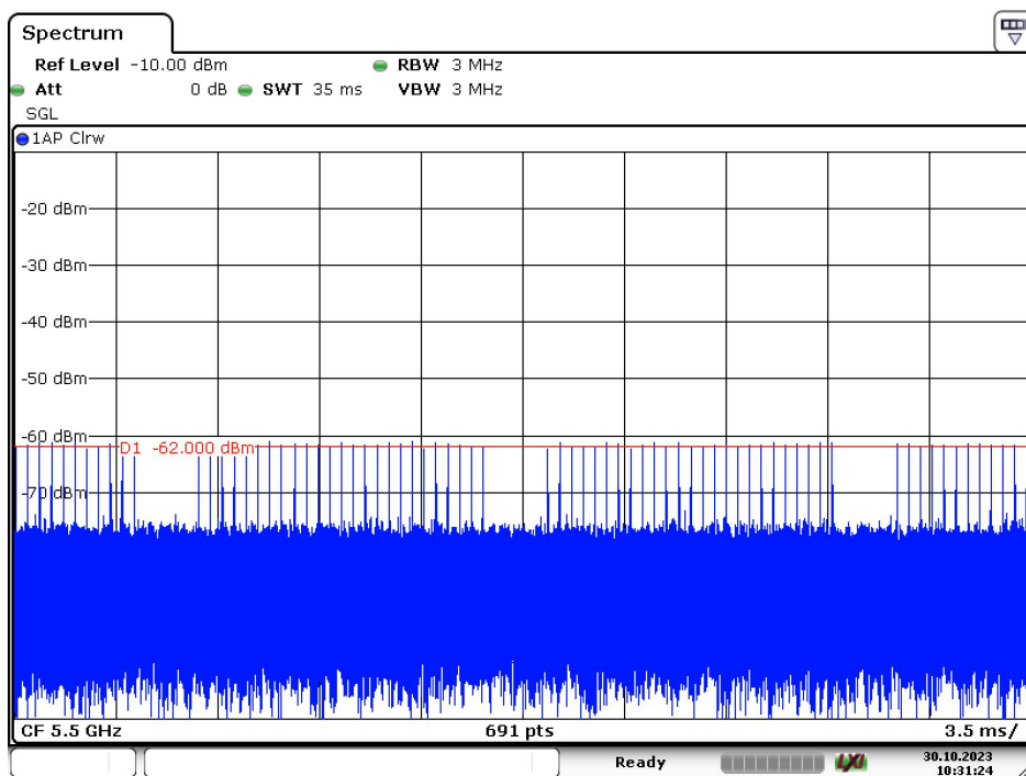
Radar Type 3 – 5500MHz
