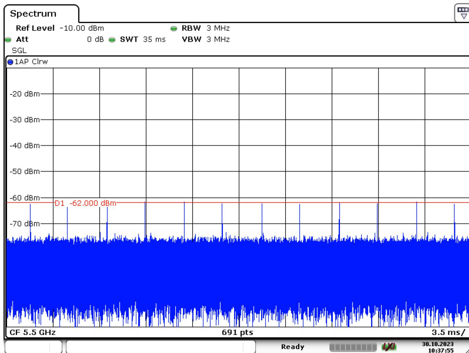
Radar Type 5 – 5500MHz
